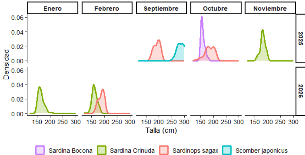
¿Figura 1: Variación temporal de la distribución de tallas en pelágicos menores
