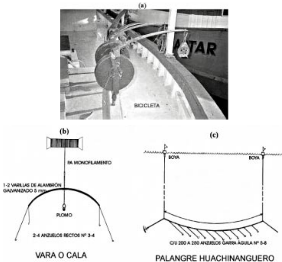
Fig. 2. Artes de pesca utilizados en la captura comercial de huachinango en el Golfo de México. (a) Bicileta; (b) Vara o Cala y (c) Palangre Huachinanguero (b y c adaptados de Oviedo et al. , 1998).
