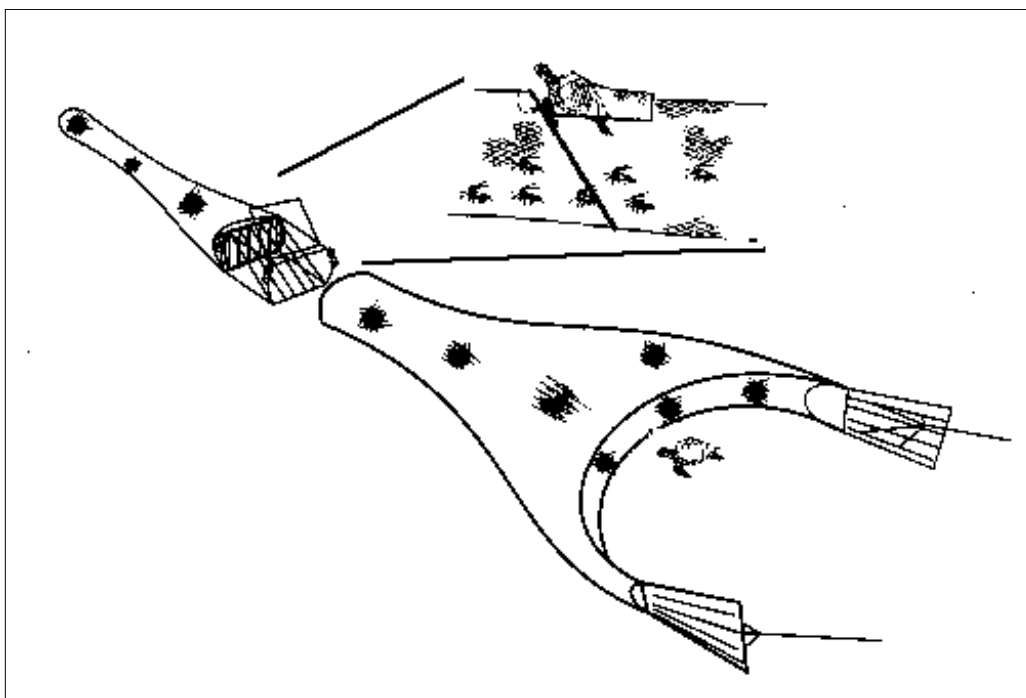
Fig. 7. Excluidores de tortugas en las redes de camarón, para evitar la mayor fuente de mortalidad de tortugas marinas.
