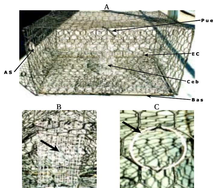
Fig. 7. Esquema de la trampa o nasa tipo Chesapeake utilizada para la captura de jaiba en la costa de Sonora. A) equipo completo de 0.6'0.6'0.4 m, B) cebadero, C) anillo selector de talla ( cull ring ). Pue=puerta, EC=entrada cónica, Ceb=cebadero, Bas=base, AS=anillo selector.
