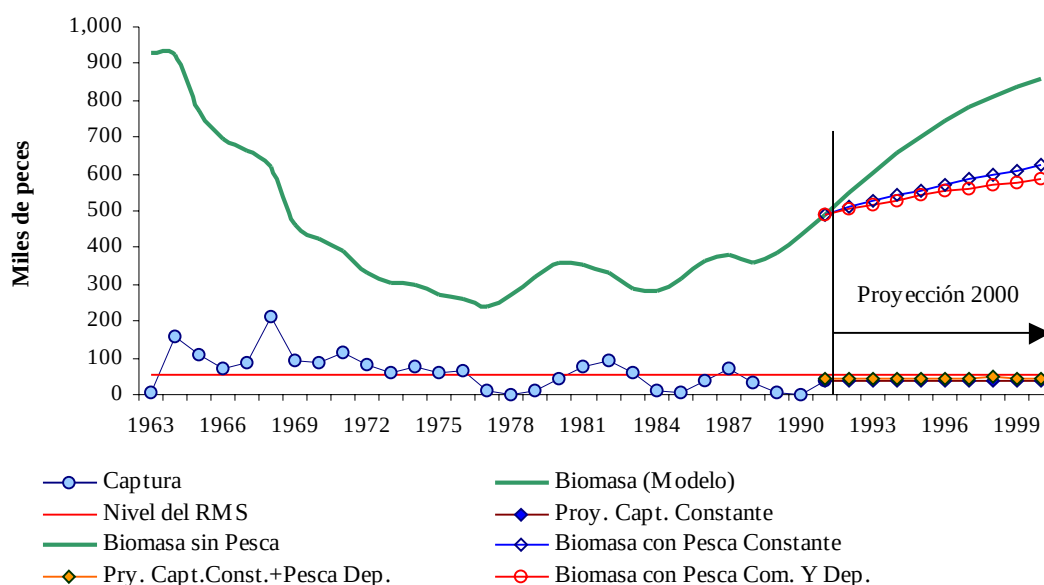
Fig. 12. Curvas de biomasa para el marlin rayado en la Zona Económica Exclusiva del Pacífico mexicano, según el modelo dinámico de Schaefer (modificado por Hilborn y Walters, 1992), y su proyección al año 2000.
