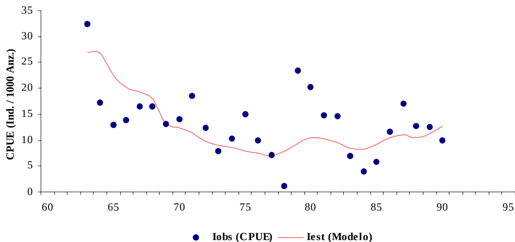
Fig. 13. Índices de abundancia estimados por el Modelo, en relación con los registrados en la pesquería, en el área representativa de la ZEE-PM, 1963-1990.
