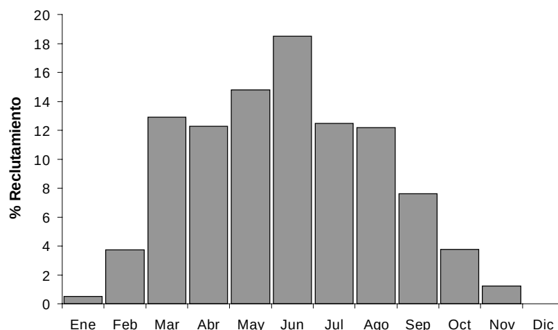
Fig. 6. Histograma del patrón de reclutamiento de la jaiba, C. bellicosus , en la pesquería de la costa de Sonora.
