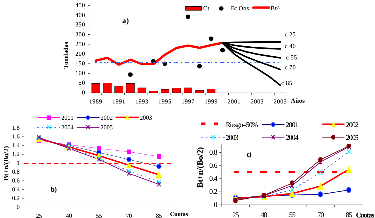
Fig. 13. a) Proyecciones de biomasa, b) Probabilidad de B_{t+n}/(Bo/2) y c) Nivel de riesgo bajo cinco diferentes cuotas de captura para la Zona III.
