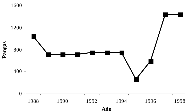
Fig. 5. Evolución del esfuerzo de pesca de sierra en Sonora.
