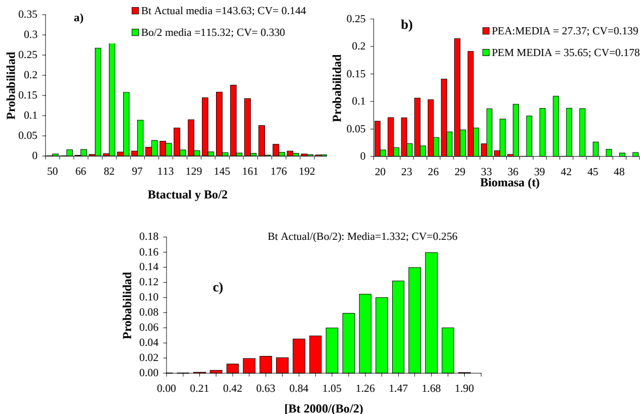
Fig. 6. a) Distribucion de probabilidades de la estimación de biomasa actual, Bo/2, b) Producción excedente actual y máxima y c) dpp del punto de referencia objetivo de la zona II.
