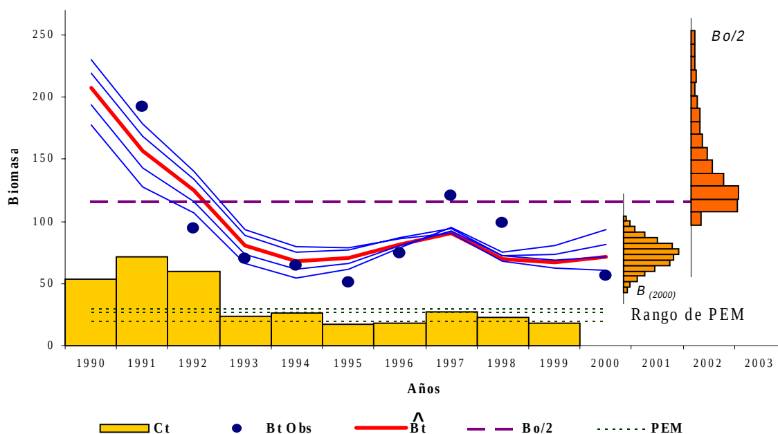
Fig. 8. Ajuste del modelo de producción excedente de Schaefer en su versión dinámica (Hilborn & Walters, 1992) a los datos de biomazas de abulón azul estimados de manera directa en la zona de la Cooperativa II.
