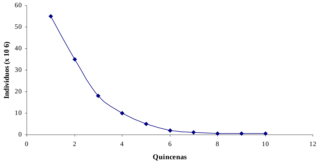
Fig. 5. Tendencia de la cohorte de D. gigas
