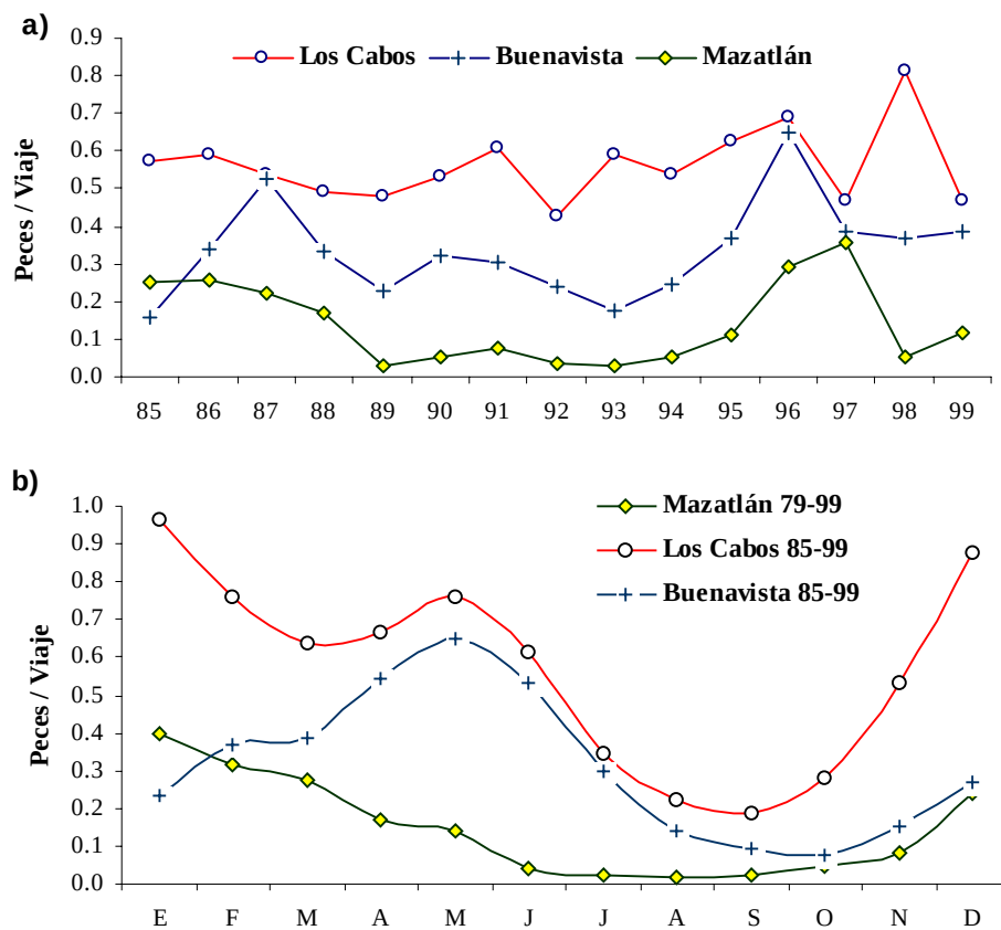
Fig. 8. a) Variación anual de las tasas de captura deportiva de marlin rayado en los principales centros turísticos del Pacífico central mexicano, y b) Media mensual.
