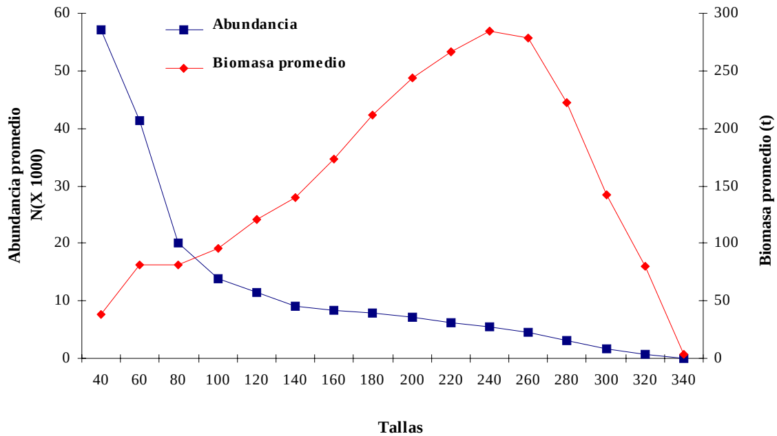
Fig. 9. Distribución de la abundancia y biomasa promedio por longitud de Sphyrna lewini para 1997.
