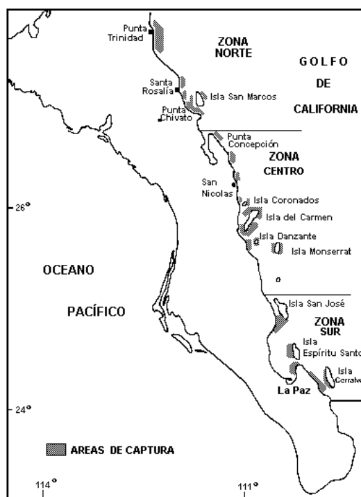
Fig. 3. Áreas de captura de I. fuscus en Baja California Sur, México.
