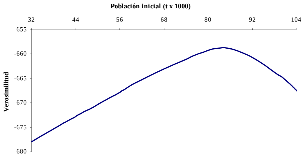
Fig. 4. Tamaño de la población de D. gigas con el modelo de flotas múltiples.
