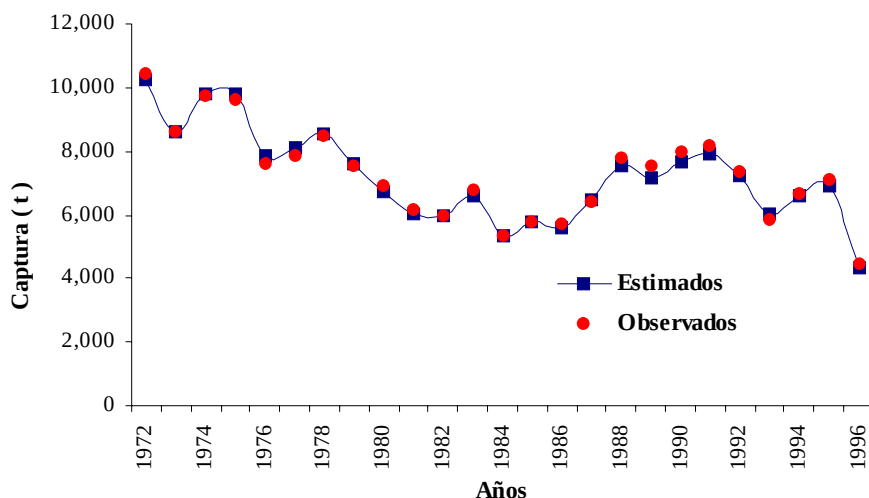
Fig. 8. Ajuste del modelo con la estructura por clases de edad de la captura, observada a partir de los muestreos mensuales realizados de 1972-1996 y estimada por el modelo.
