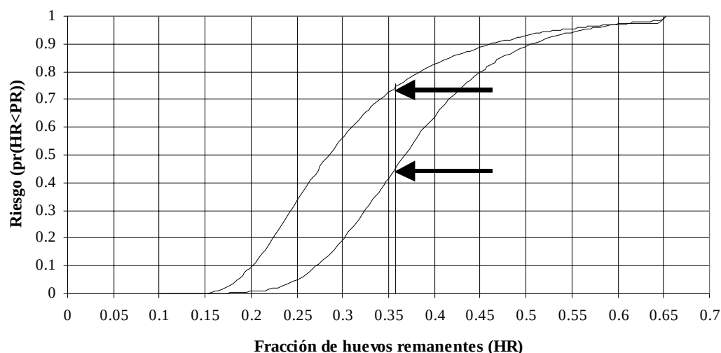
Fig. 10. Envoltura del riesgo de que la fracción de huevos remanentes sea menor que el punto de referencia. Si se selecciona 35% (0.35) como punto de referencia, el riesgo de que HR sea menor será de entre 41.7 y 72.7%, según la talla mínima de captura.
