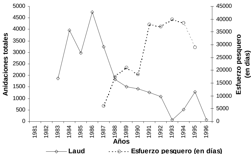
Fig. 3. Decremento del número de anidaciones en la playa de Mexiquillo e incremento en el esfuerzo pesquero en Chile.
