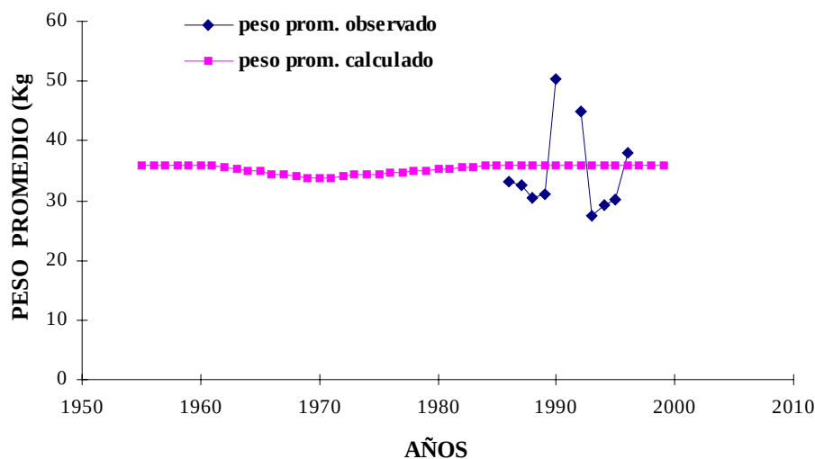
Fig. 8. Ajuste del modelo con desfaseamiento, utilizando el peso promedio observado y el peso promedio calculado.
