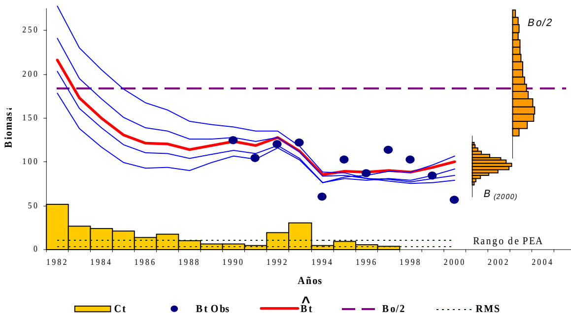
Fig. 6. Ajuste del modelo de producción excedente de Schaefer en su versión dinámica (Hilborn y Walters, 1992) a los datos de biomاسas de abulón amarillo estimadas de manera directa en la zona de la Cooperativa I.
