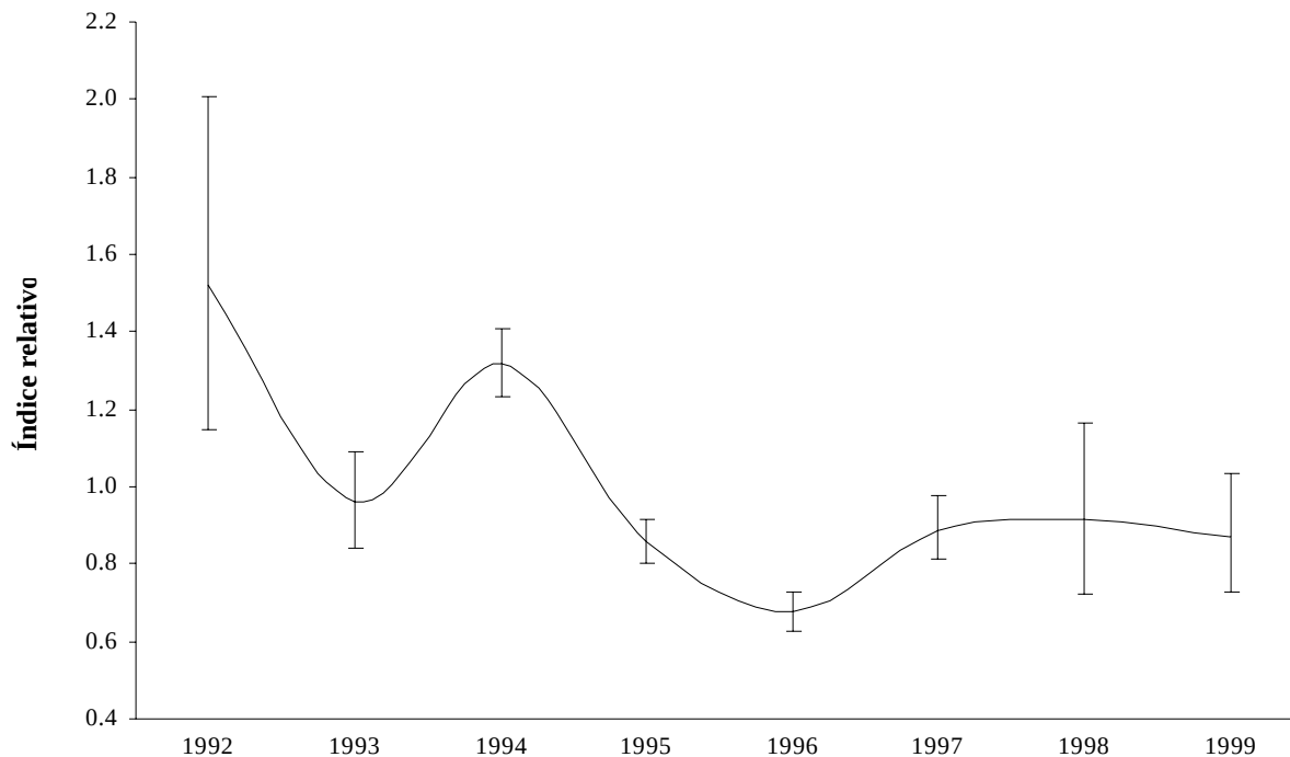
Fig. 10. Tendencia del índice de abundancia estandarizado para el atún aleta amarilla e intervalos de confianza de 95%. Valores relativos al promedio de la serie 1992-1999 (Índice relativo = 1.0). Flota internacional en el Golfo de México. Resultados preliminares.
