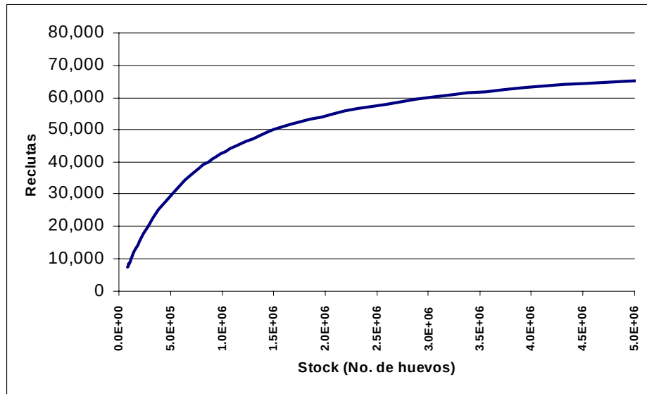
Fig. 9. Relación Stock-reclutamiento con a partir de B_0 = 3'000,000 , R_0 = 60,000 , z = 0.55 . Los datos observados son la densidad observada de tortugas de la clase de edad (24 cm) en Río Lagartos extrapolada a toda la península, de los años 1997, 98 y 99 los círculos consideran el número de huevos de un año antes y los cuadros de 2 años antes.
