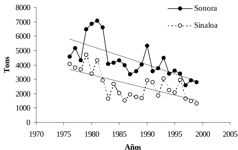
Fig. 5. Series de producción de tiburón de los estados de Sonora y Sinaloa. La línea continua representa la tendencia relativa.
