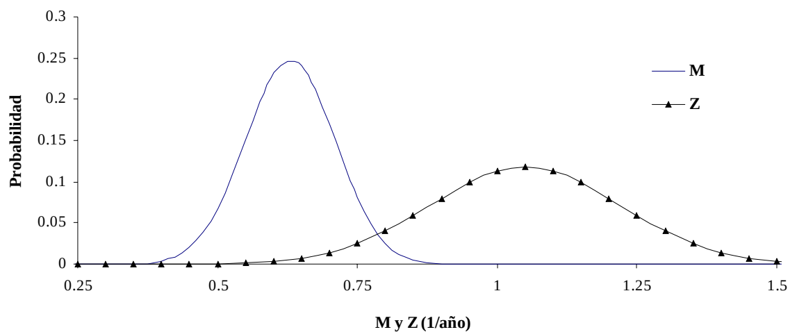
Fig. 6. Distribución de probabilidad de las estimaciones de mortalidad natural (M) y total (Z).
