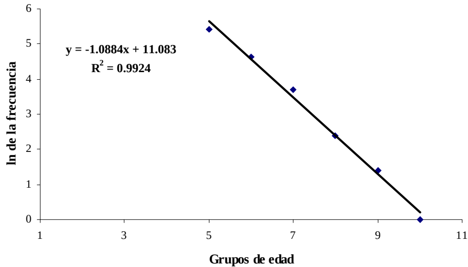
Fig. 4. Estimación de la mortalidad total para pez vela en el Pacífico mexicano, por el método de curva de captura.
