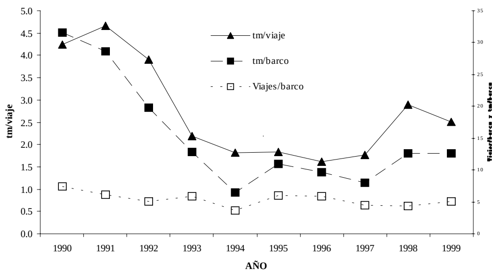
Fig. 7. Captura por unidad de esfuerzo de pez espada (1996: datos preliminares enero-junio). Flota agallera mexicana.
