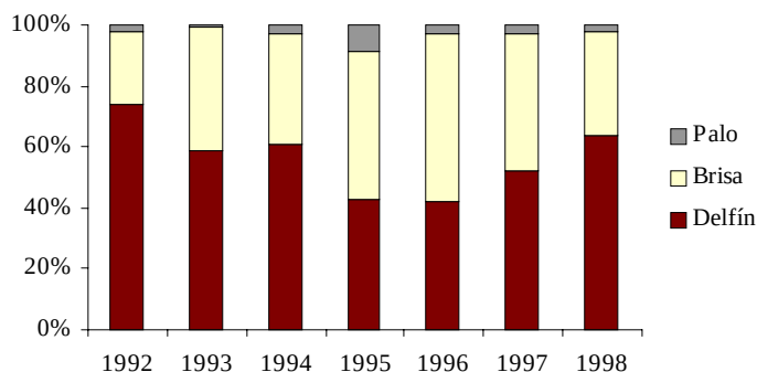
Fig. 4. Porcentaje de lances de la flota mexicana, asociados a delfín, brisa y palos.
