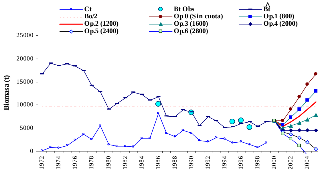
Fig. 7. Proyecciones de biomasa de erizo rojo en Baja California, México, bajo diferentes opciones de captura (t) con base en el Modelo de Schaefer.
