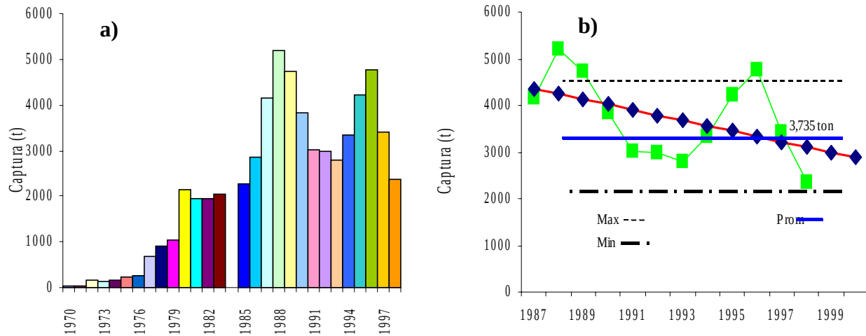
Fig. 3. Captura histórica de Mugil cephalus (a) y tendencia en los últimos 12 años (b). Laguna Madre, Tamaulipas.
