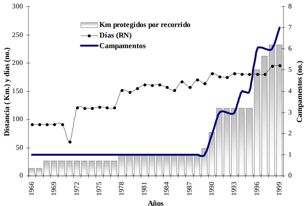
Fig. 2. Evolución del esfuerzo invertido en la protección. Los días indican la duración de las actividades en el campamento de Rancho Nuevo, Tamps. La distancia indica el intervalo que se protege en cada uno de los recorridos, según el número de campamentos instalados. El número de recorridos promedio por día es de tres.
