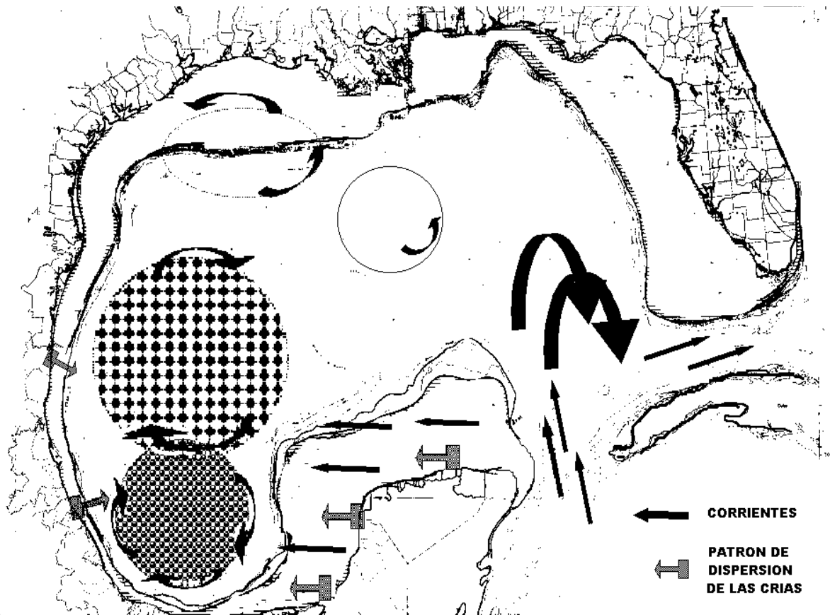
Fig. 2. Corrientes marinas que afectarían el patrón de dispersión de las crías de tortuga nacidas en Rancho Nuevo según Collard y Ogren, (1990). Se aplica el mismo modelo para las crías nacidas en la península de Yucatán, que se moverían hacia el centro del Golfo de México quedando dentro de los giros achurados.
