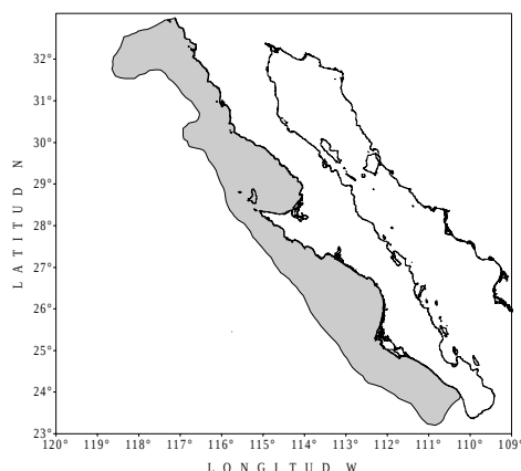
Fig. 1. Area de distribución del bacalao negro en las costas mexicanas.
