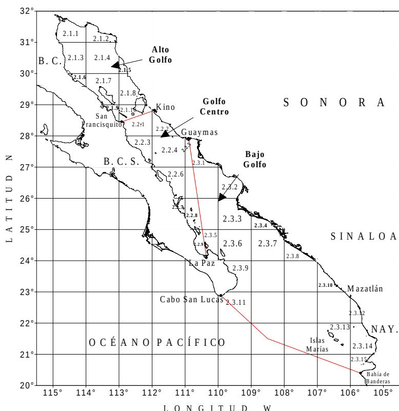
Fig. 2. Diversidad de especies de peces marinos de ornato, con base en la regionalización del Golfo de California.
