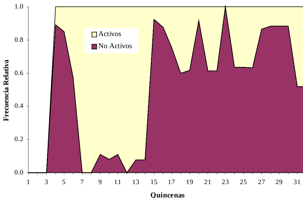
Fig. 8. Variación temporal de la madurez de Dosidiscus gigas
