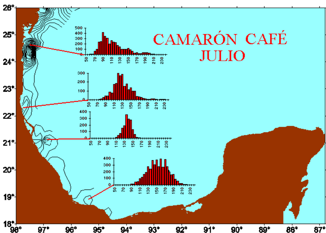
Fig. 1. Rendimiento (Kg/hora de arrastre) y tallas (longitud total en mm) de camarón café, de cruceros en época de veda en 1997.
