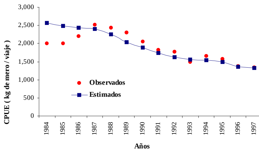
Fig. 9. Ajuste del modelo con la captura por unidad de esfuerzo de la flota mayor mexicana (CPUE flota mayor), observada y estimada por el modelo, durante 14 años (1984 – 1997).
