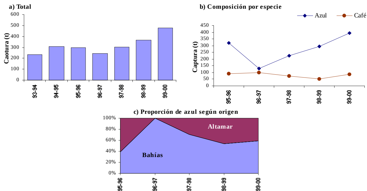
Fig. 3. Tendencia de la captura de camarón registrada para la zona del Alto Golfo de la temporada 1988-1989 a la 1999-2000: a) captura total; b) por especies y c) según origen.
