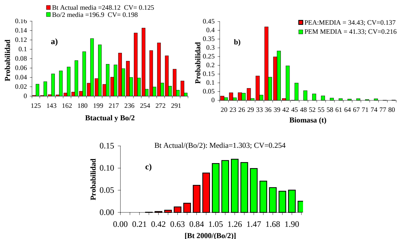
Fig. 4. a) Distribucion de probabilidades de la estimación de biomasa actual, Bo/2, b) Producción excedente actual y máxima y c) dpp del punto de referencia objetivo.
