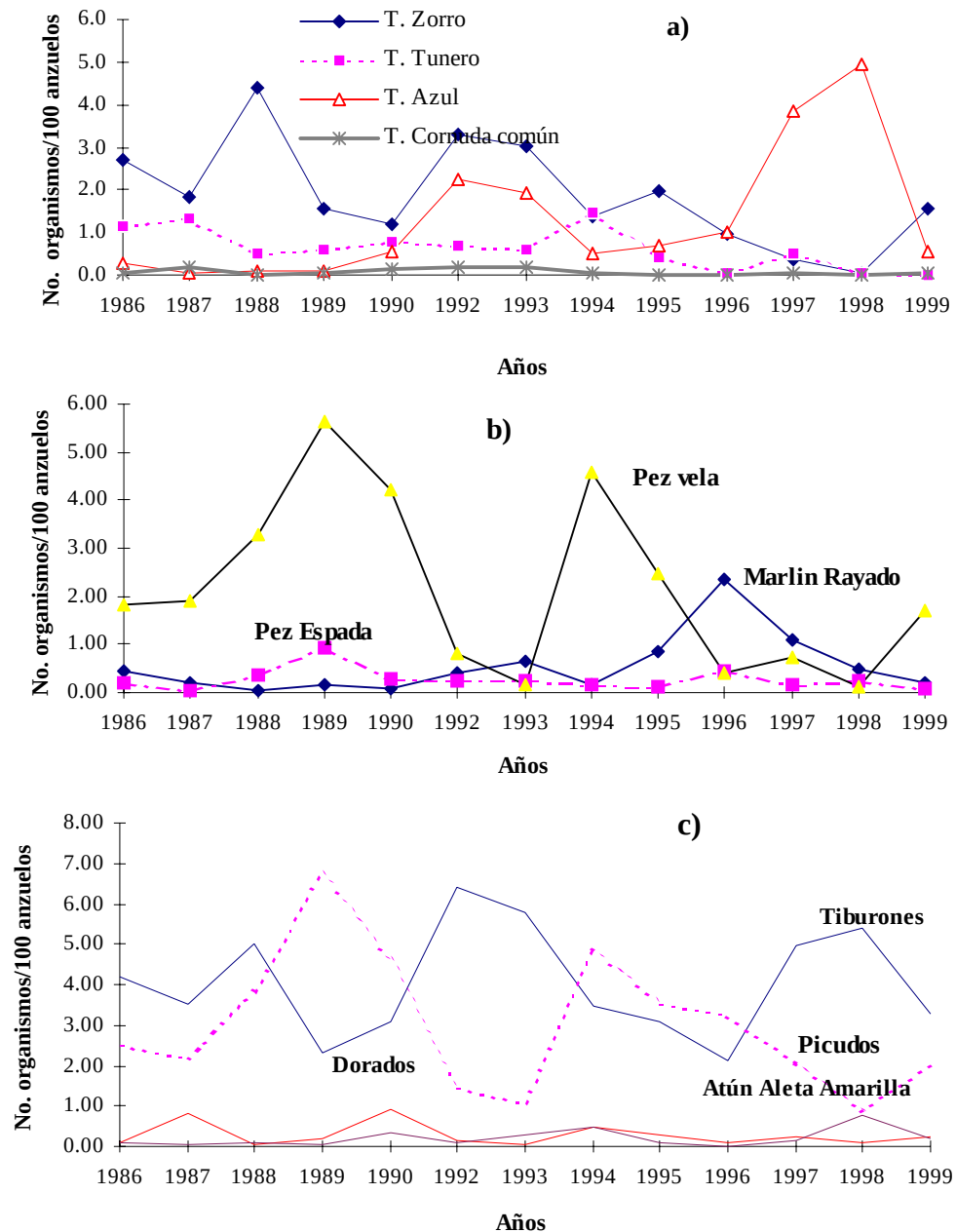
Fig. 3. Captura por unidad de esfuerzo de la flota palangrera oceánica, durante el periodo 1986-1999. a) tiburón, b) picudos y c) pelágicos mayores.
