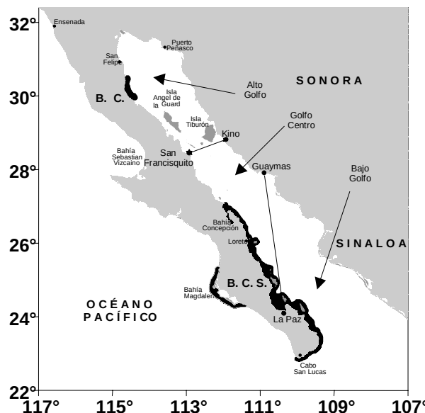
Fig. 1. Zonas de captura de especies marinas de ornato en el Golfo de California y Pacífico norte.
