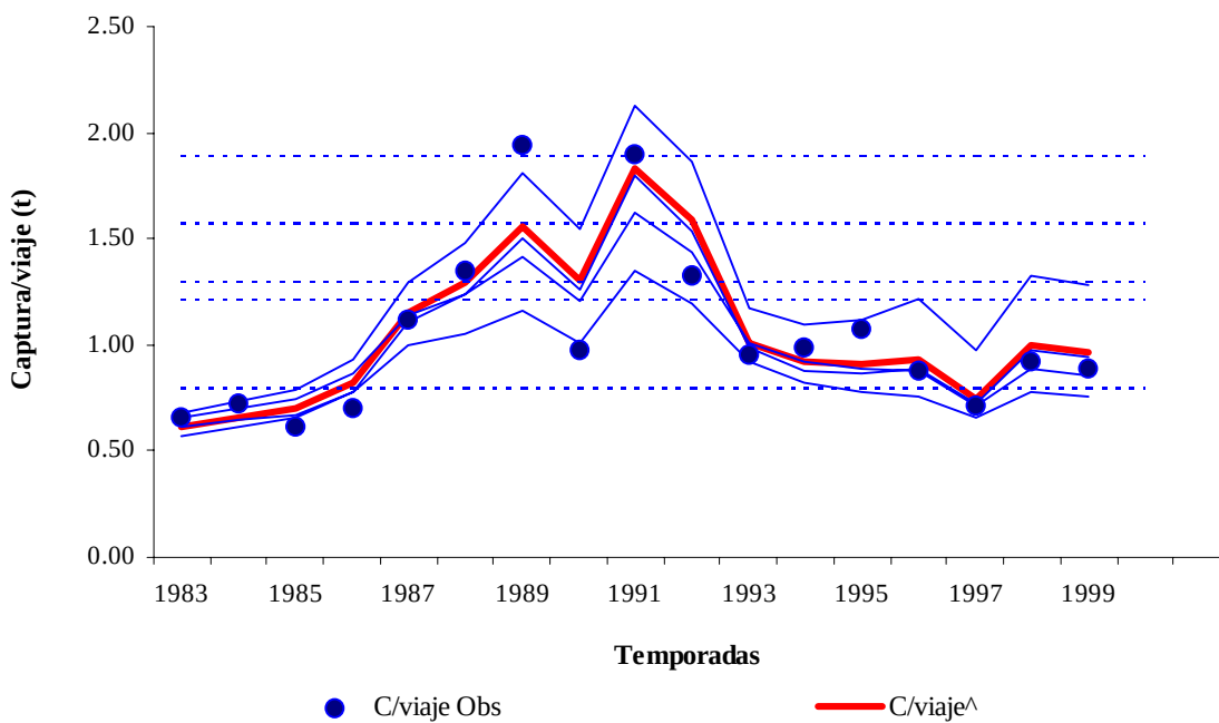
Fig. 20. Ajuste del modelo dinámico de biomasa de Schaefer a los datos de captura/viaje de camarón café, F. californiensis , descargado en la zona de Mazatlán, Sin. durante las temporadas 1983-84 a 1999-2000.
