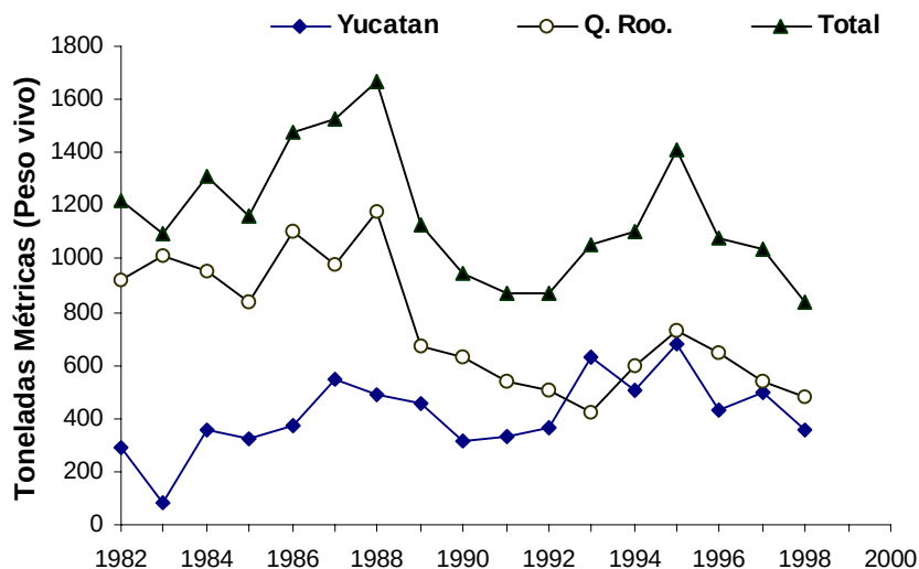
Fig. 1. Capturas de langosta espinosa en la Península de Yucatán, periodo 1982-1998.
