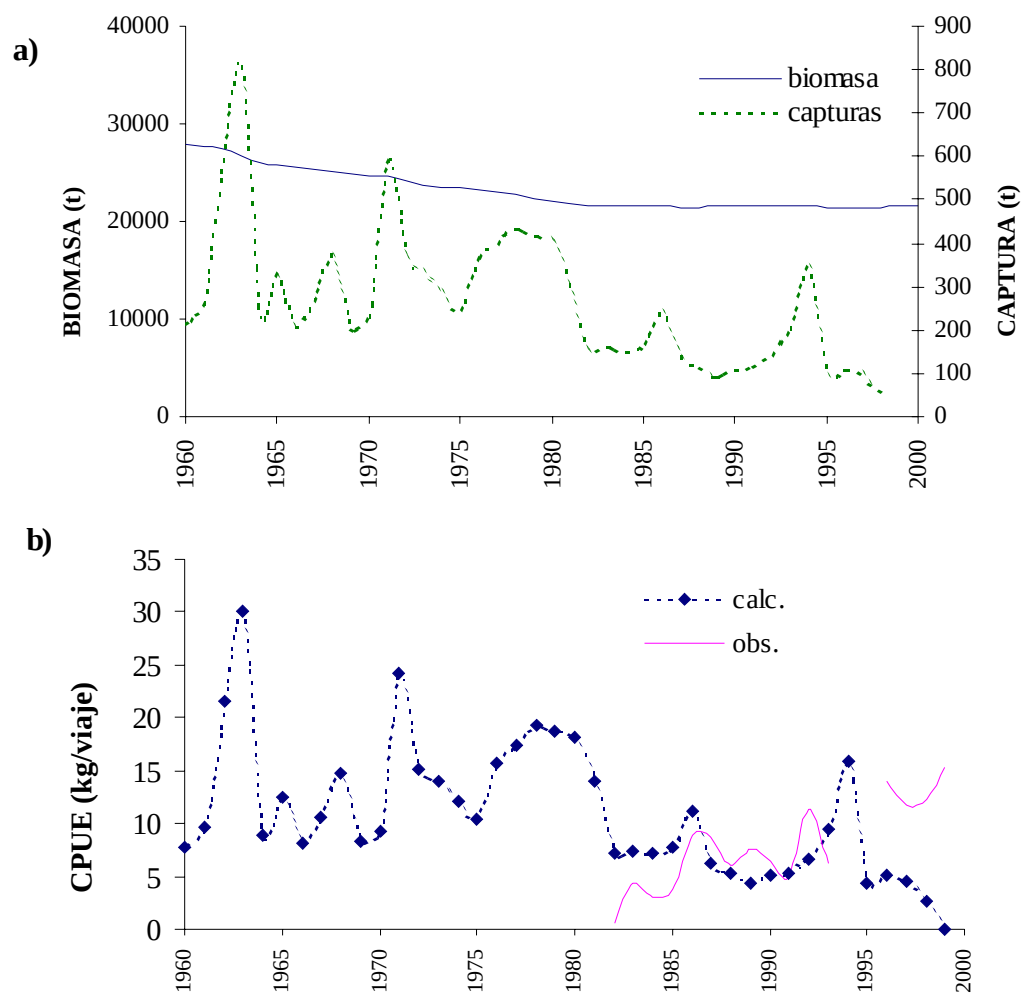
Fig. 9. a) Biomasa calculada para huachinango por el modelo de Deriso o modelo de diferencia con retraso, y b) Validación de la captura por unidad de esfuerzo observada y la calculada por el método de Deriso.
