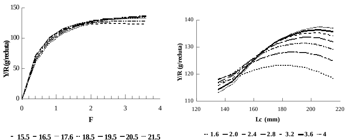
Fig. 4 Resultados de la simulación con modelo de rendimiento por recluta de Beverton y Holt, variando la talla de primera captura y la tasa de mortalidad por pesca.
