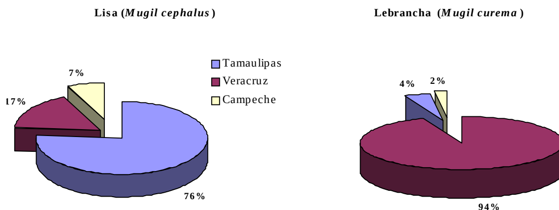
Fig. 1. Proporción promedio de la captura de lisa y lebrancha a nivel nacional, 1990-1999.
