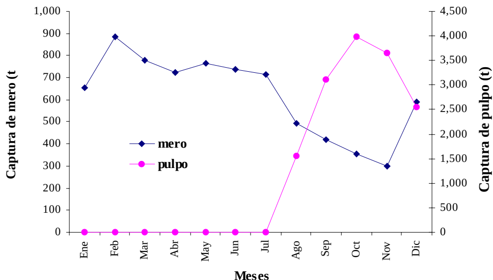
Fig. 3. Comportamiento mensual de la captura promedio de mero y pulpo obtenida por la flota mayor y artesanal mexicana que operan en el Banco de Campeche (1996-1998) (SEMARNAP, Delegación Federal en Yucatán).
