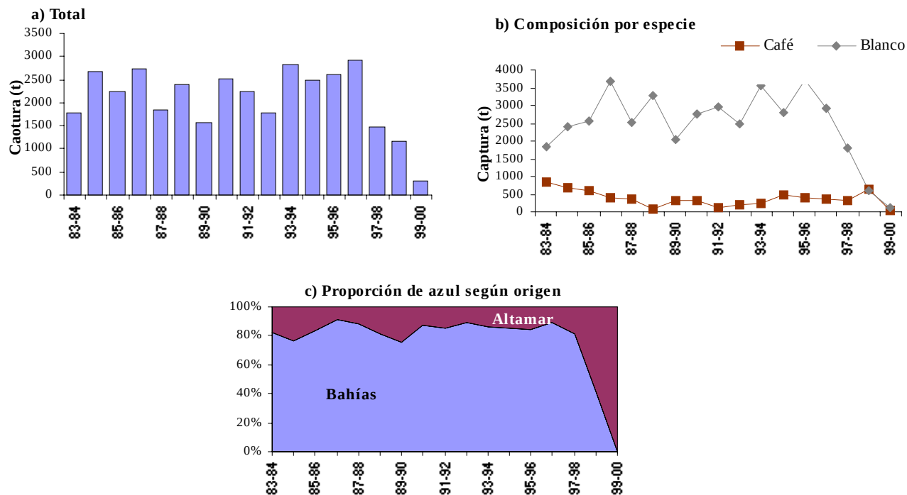
Fig. 5. Tendencia de la captura de camarón registrada en Salina Cruz, Oax. de la temporada 1988-1989 a la 1999-2000: a) captura total; b) por especies y c) según origen
