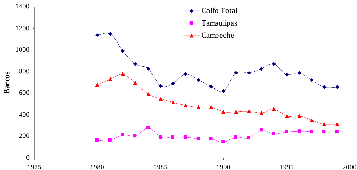
Fig. 5. Evolución del número de barcos camaroneros en el Golfo de México y en los estados de Tamaulipas y Campeche.
