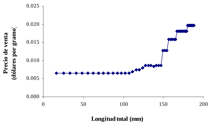
Fig. 17. Variación de precio (dólares por gramo) de camarón blanco de acuerdo con la talla.
