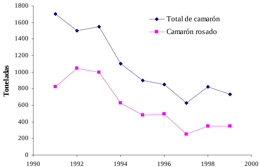
Fig. 12. Tendencias históricas de las capturas de camarón en el Puerto de Campeche.
