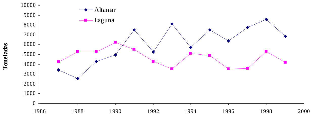
Fig. 7. Captura de camarón por sistema en el estado de Tamaulipas.
