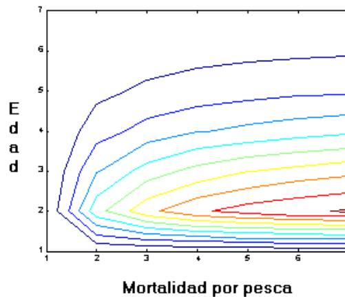
Fig. 6. Modelo de Rendimiento por Recluta.
