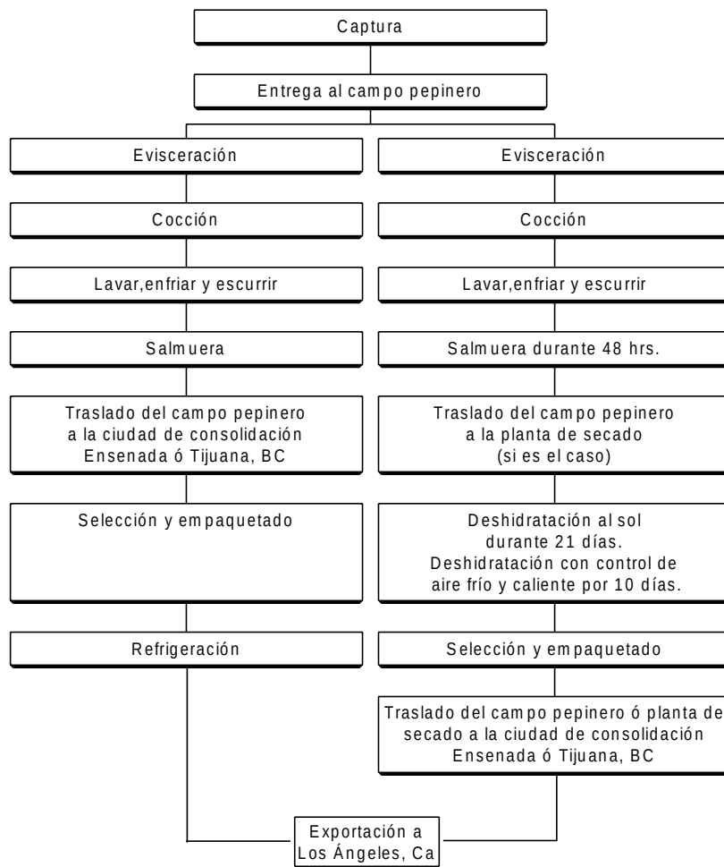
Fig. 5. Diagrama de flujo de los procesos que se aplican a I. fuscus en Baja California, para obtener las presentaciones de exportación (Ramírez-Soberón, 2000b).
