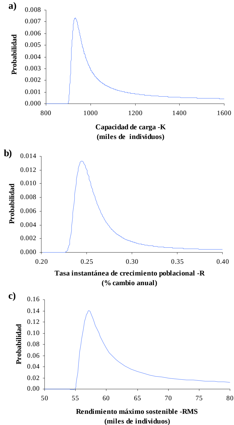
Fig. 11. Probabilidades posteriores de Bayes para la capacidad de carga (a), la tasa instantánea de crecimiento poblacional (b), y el rendimiento máximo sostenible (c), para la pesquería de marlin rayado en el Pacífico mexicano.
