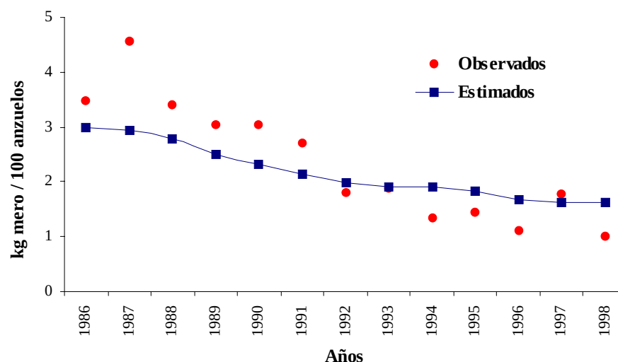
Fig. 11. Ajuste del modelo con los índices de la abundancia (IAcrucero) observados a través de 28 cruceros de investigación durante 14 años (1986-1998).
