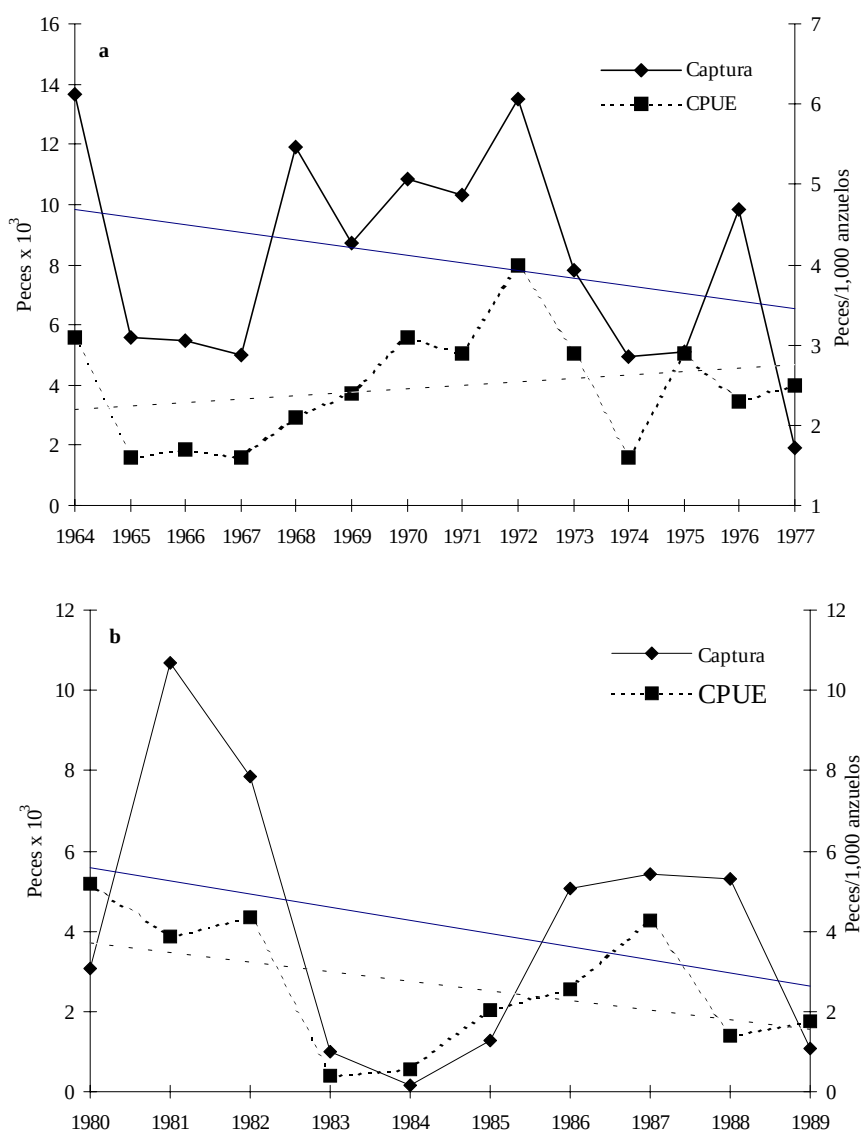
Fig. 5. Captura de pez espada, CPUE y sus tendencias. (a) Flota palangrera japonesa, área núcleo al sur de Baja California. (b) Flota palangrera de conversión, ZEEM.
