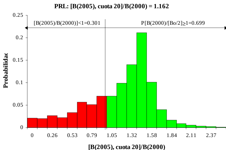
Fig. 19. Distribución posterior de probabilidad del Punto de Referencia Limite de abulón en la zona concesionada a la cooperativa II; proyección de biomasa al 2005 con una cuota de 20 t. El riesgo está representado por las barras oscuras a la izquierda de la línea vertical.
