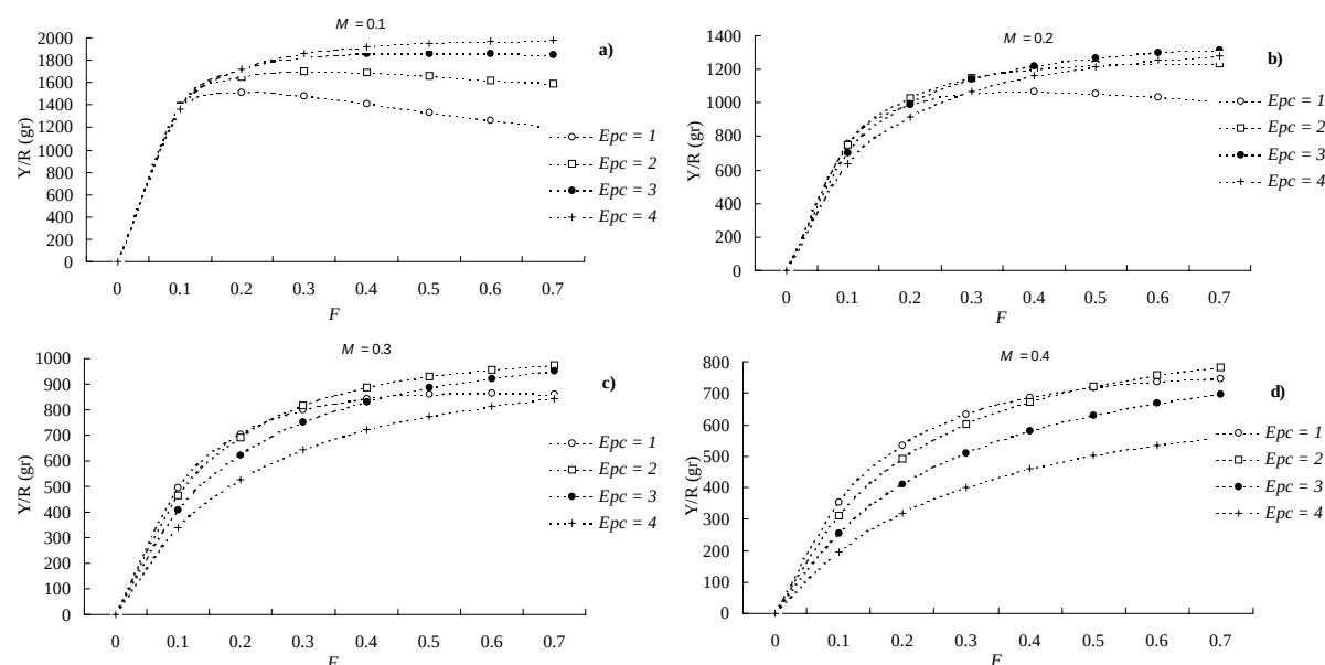
Fig. 5. Estimación del Rendimiento por Recluta de R. terraenovae , variando M desde 0.1 hasta 0.4 y F = 0.46 .
