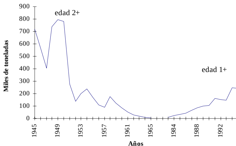
Fig. 5. Biomasa de sardina Monterrey de edad 2+ para los años 1945-1965 (MacCall, 1979) y edad 1+ para 1983-1995 (Deriso et al. , 1996).
