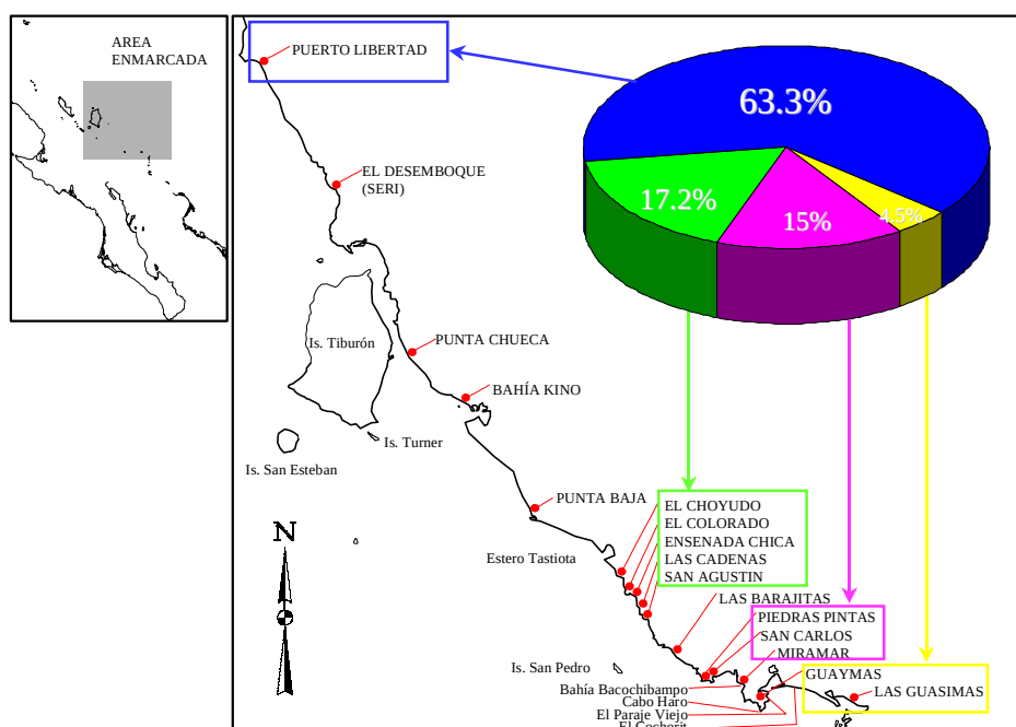
Fig. 2. Localidades de captura de sierra en el Golfo de California.
