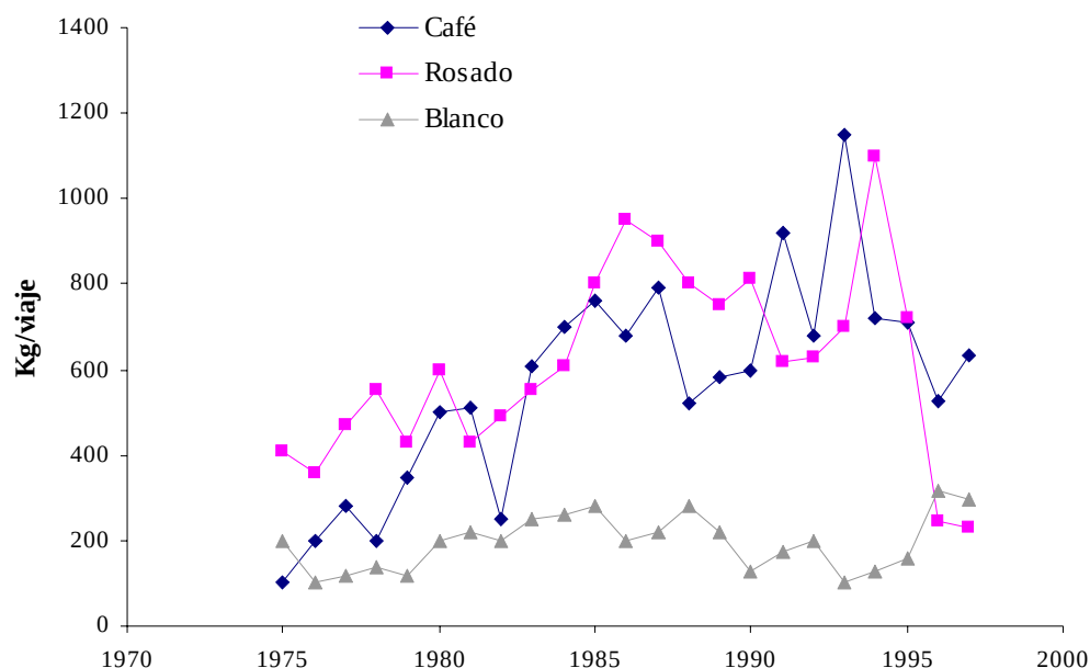
Fig. 11. Comportamiento de la captura por unidad de esfuerzo (viajes) de las tres especies registradas por la flota camaronera de Ciudad del Carmen, Camp.
