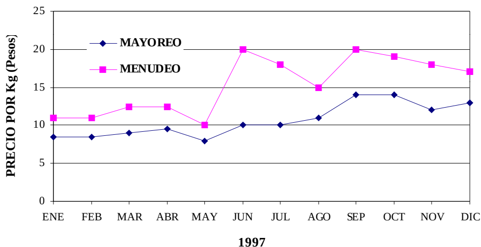
Fig. 6. Precios de playa del pez vela en Manzanillo, Col.
