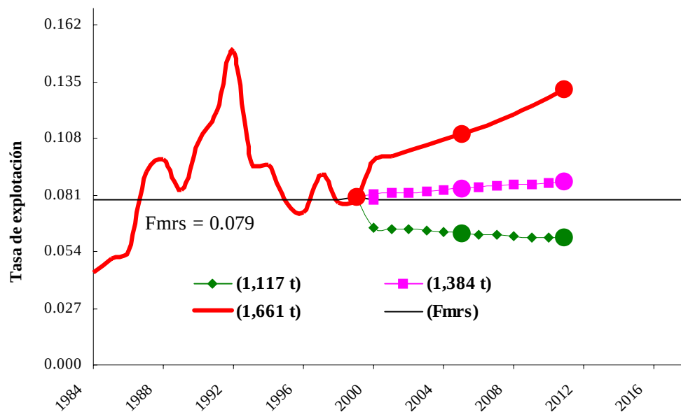
Fig. 7. Comportamiento y proyecciones de la tasa de explotación de la pesquería de huachinango ( Lutjanus campechanus ), en el Banco de Campeche, ante diferentes cuotas de captura.
