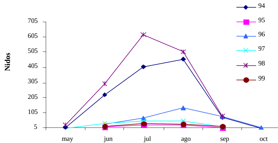
Fig. 4. Variación estacional de hembras de tortuga blanca, anidando en la playa de Lechuguillas, Veracruz, en las temporadas de 1994 a 1999.
