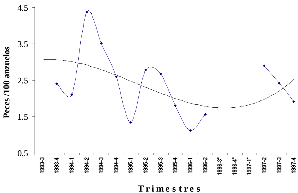
Fig. 9. Tendencia de la tasa de captura nominal para el atún aleta amarilla. Flota palangrera mexicana.
