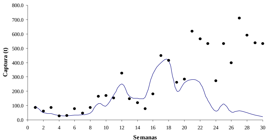
Fig. 6. Reconstrucción y pronóstico de las capturas de D. gigas .
