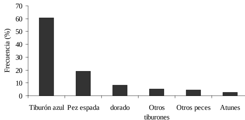
Fig. 9. Composición de la captura durante 1998-2000, por la flota palngretera.
