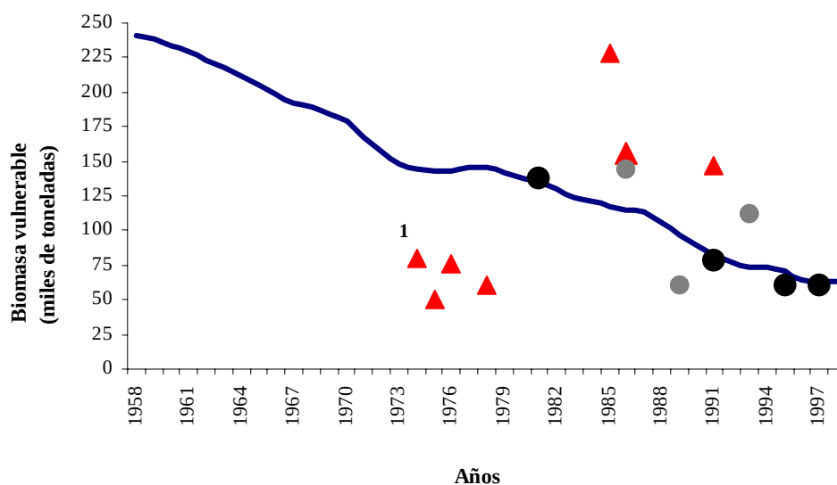
Fig. 7. Tendencia de la biomasa vulnerable del stock de mero estimada por el modelo (1958-1998). Los puntos negros son evaluaciones realizadas por otros autores que caen dentro de las estimaciones de este modelo; los puntos grises se pueden considerar estimaciones cercanas y los triángulos son estimaciones que distan de la evaluación actual. 1) González y Ramis (1974); 2) González y Ramis (1975); 3) Klima (1976); 4) Buesa (1978); 5) Doi et al. (1981); 6) Arreguín (1985) 7) Fuentes y Contreras (1986); 8) Seijo (1986); 9) Valdés et al. (1989); 10) Zetina et al. (1996); 11) Valdés et al. (1991); 12) Contreras et al. (1993); 13) Moreno et al. (1995) y 14) Moreno et al. (1997).
