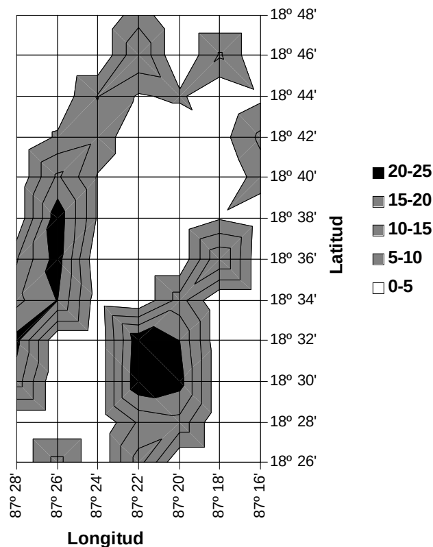
Fig. 3. Distribución de la biomasa de pulpa de caracol ( Strombus gigas ) en el sistema simulado para Banco Chinchorro, Quintana Roó.
