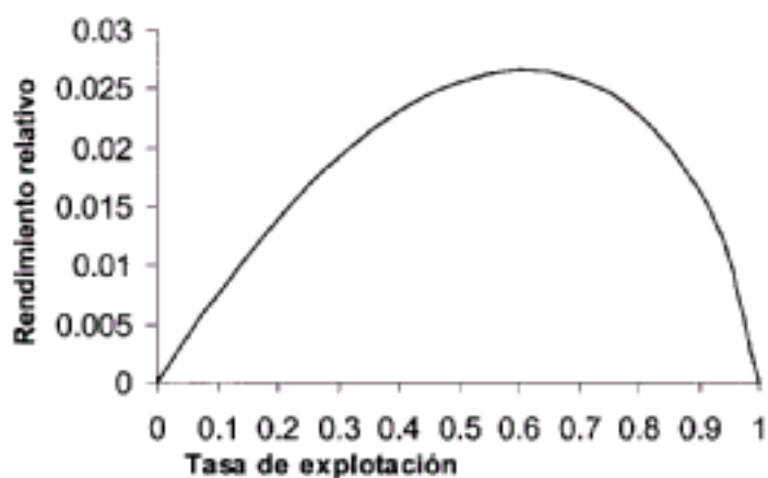
Fig. 4. Rendimiento relativo por recluta de lisa en Sinaloa.
