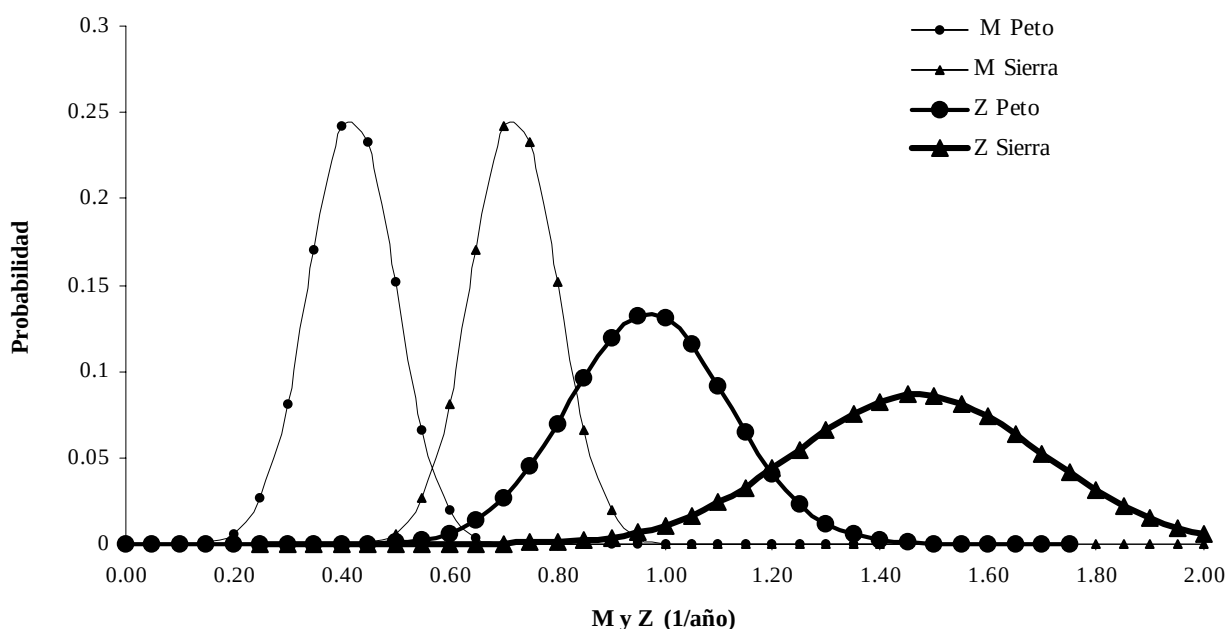
Fig. 4. Distribución de probabilidad de los estimados de M y Z para peto y sierra.
