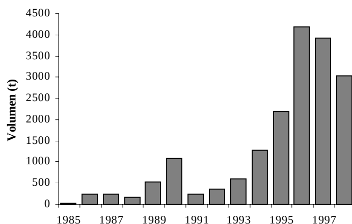
Fig. 8. Producción de jaiba en el estado de Sonora (1985-1998).
