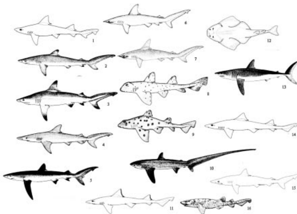
Fig. 1. Tiburones de importancia capturados en la pesca artesanal del Golfo de California.
