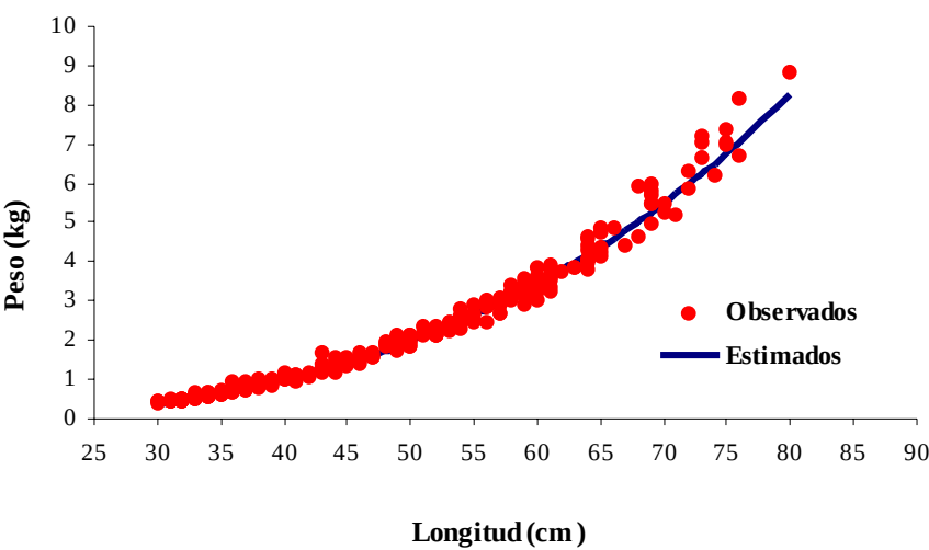
Fig. 5. Relación peso-longitud del mero en el Banco de Campeche.
