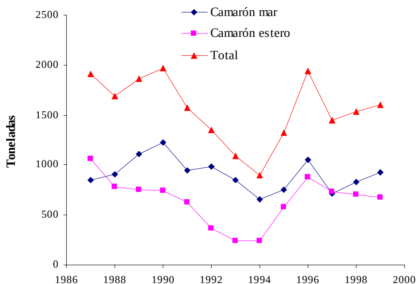
Fig. 9. Captura en toneladas de camarón de altamar y esteros en el estado de Veracruz.
