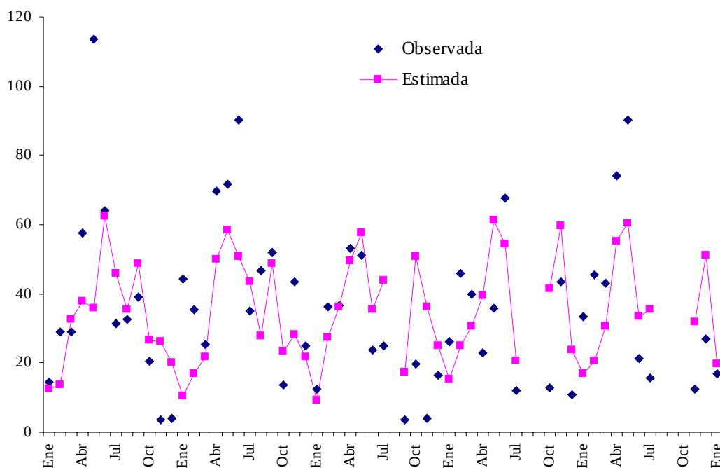
Fig. 27. Ajuste del modelo a capturas de Contoy
