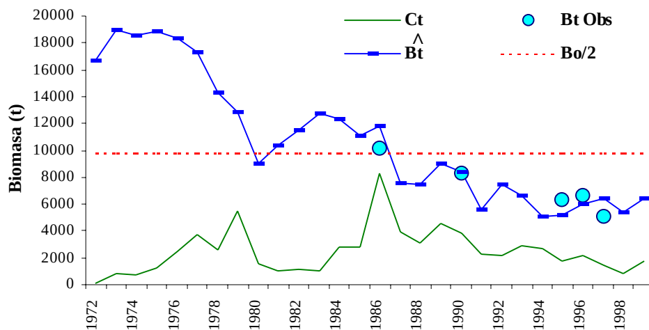
Fig. 2. Curva de biomasa estimada con el modelo de Schaefer para los datos de biomasa del erizo rojo en Baja California, México, durante el periodo de capturas 1972-2000. La biomasa estimada ( B_t ) es la representación determinística con la mejor combinación de parámetros del modelo.
