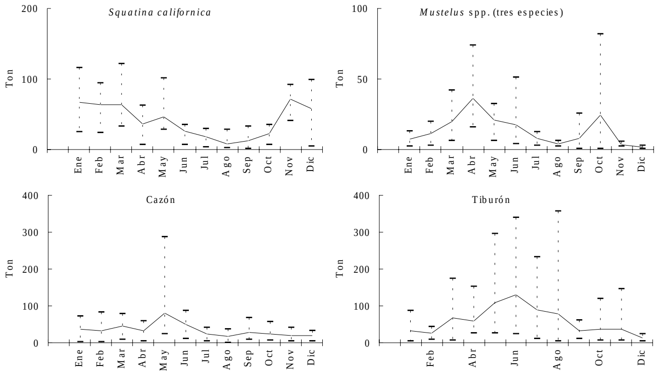
Fig. 4. Producción estacional de tiburón (por categoría) en Sonora. La línea continua representa el promedio de 1993 a 1999. Las líneas verticales representan los intervalos.
