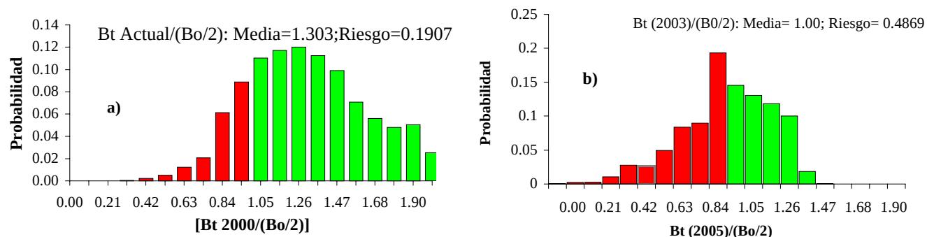
Fig. 10. Distribución posterior de probabilidades de la tasa Bt actual/ (Bo/2) y B_{t+n}/(Bo/2) de la zona I, con una cuota de 55 t.
