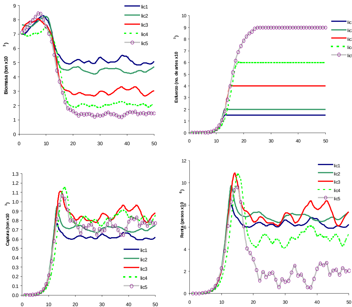
Fig. 4. Simulación con diferentes niveles de esfuerzo aplicado a la pesquería de la presa Aguamilpa, Nayarit.
