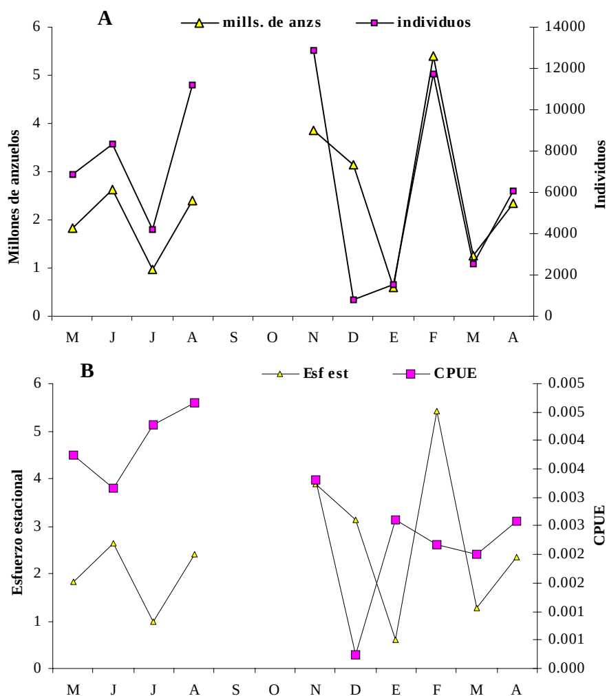
Fig. 6. Captura mensual de bacalao negro, entre mayo de 1997 y abril de 1998. A) miles de organismos y esfuerzo estandarizado, (B) esfuerzo contra CPUE.
