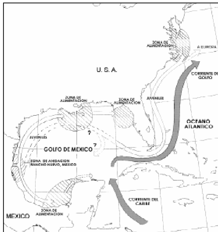
Fig. 1. Distribución geográfica de la tortuga lora L. kempi y posibles rutas migratorias. Figura adaptada de Márquez et al. , en prensa.
