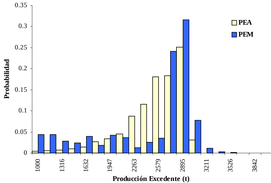
Fig. 6. Distribución de probabilidad de la producción excedente máxima (PEM) y producción excedente actual (PEA) de 1999, de la pesquería del erizo rojo de Baja California, México.
