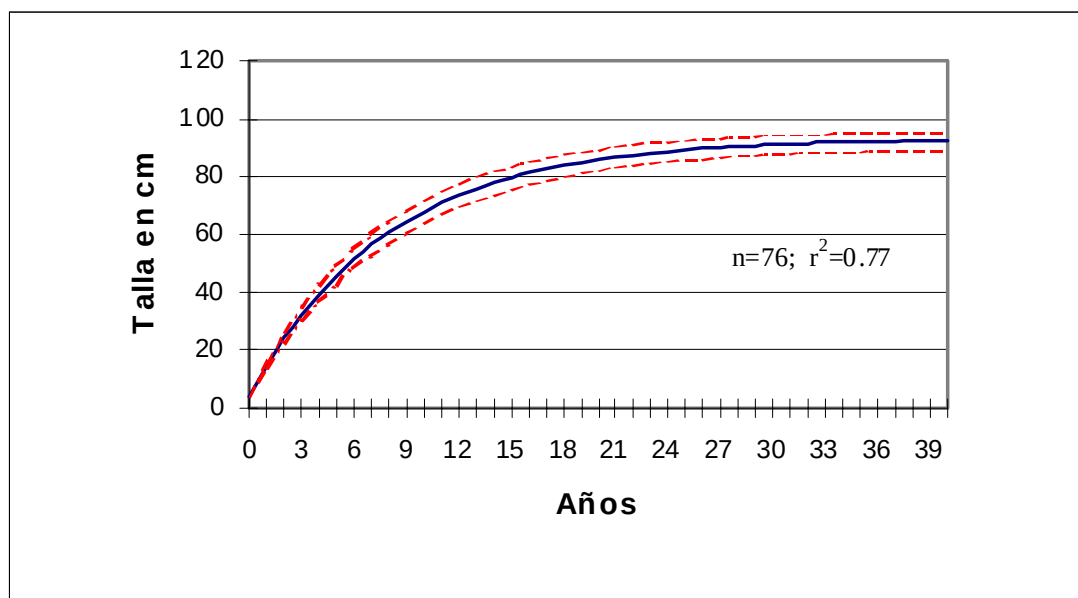
Fig. 4. Modelo de crecimiento de tortugas de carey capturadas frente a las playas de la Reserva de Río Lagartos (poner una ecuación para la curva?).
