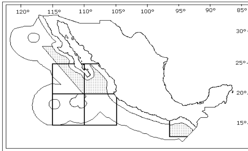
Fig. 10. Zona Económica Exclusiva del Pacífico Mexicano, franja de exclusión de 50 millas, polígonos de exclusión para la flota palangrera definidos por Acuerdo Regulatorio de 1887; área índice, y área total, según Squire y Au (1990).
