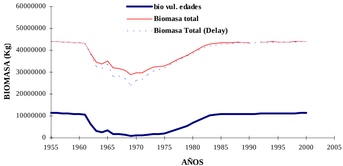
Fig. 9. Biomاسas totales y biomasa vulnerable estimada por los modelos estructurado y con desfaseamiento.
