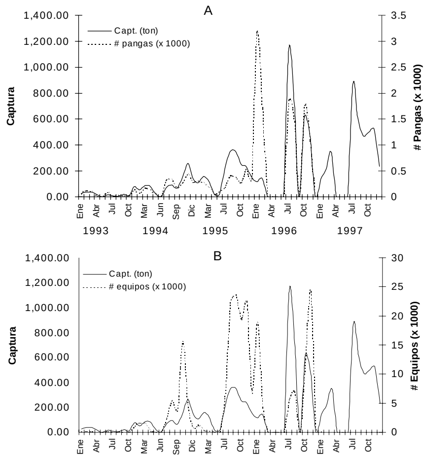
Fig. 2. Captura y esfuerzo de la pesquería de jaiba en el estado de Sonora, entre 1993 y 1998. A) por pangas, B) por equipos (trampas).
