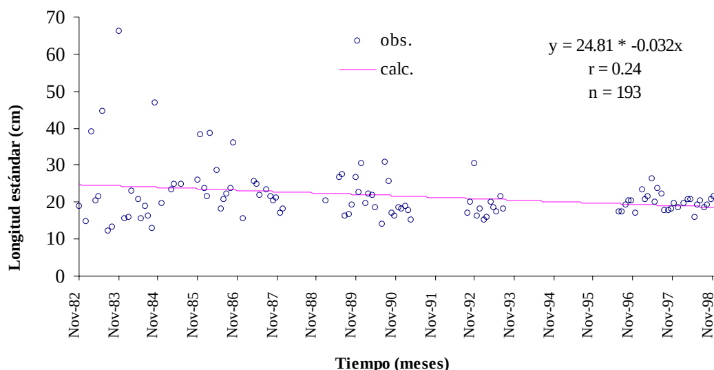
Fig. 8.- Regresión lineal con los valores originales de talla promedio del huachinango Lutjanus peru .
