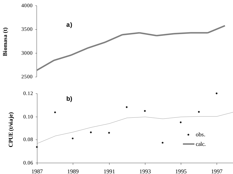
Fig. 10. Valores estimados para a) la biomasa poblacional y b) CPUE, mediante el modelo de Schaefer ajustado a los datos de la pesquería de huachinango registrada en La Cruz de Hunacastle, Nay.
