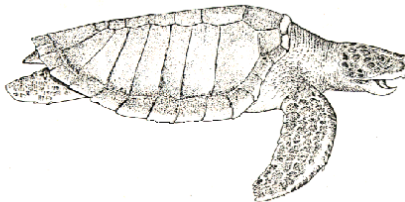
Fig. 1. Tortuga golfina, Lepidochelys olivacea .
