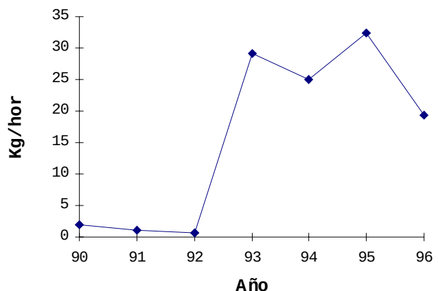
Fig. 4. Índice de abundancia anual de sardina Monterrey. Captura por hora de arrastre en el Golfo de California. (Tomada de Cisneros-Mata et al. , 1997).
