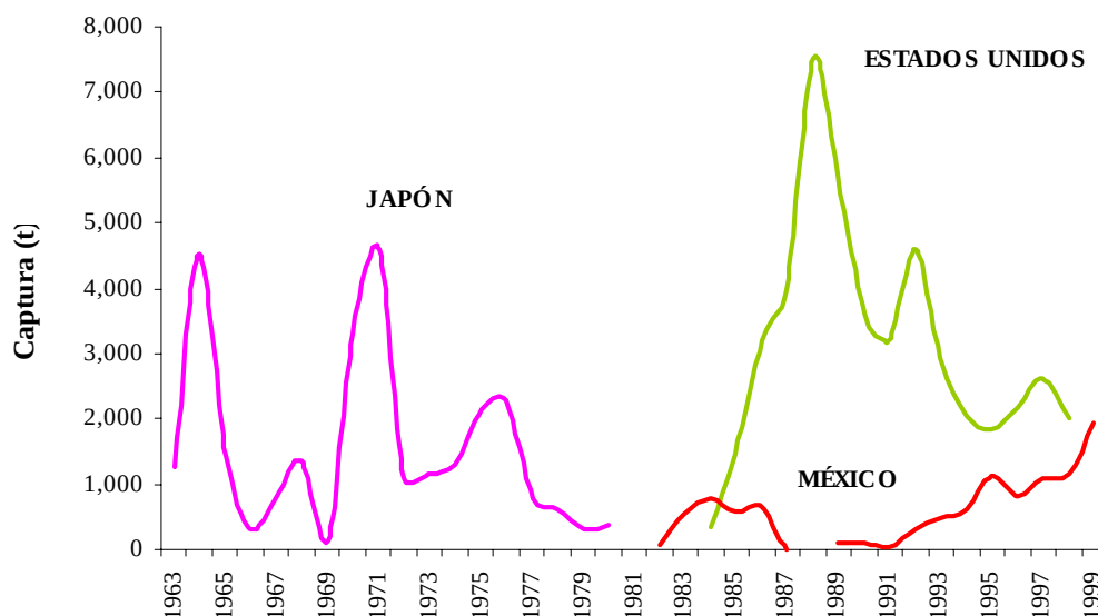
Fig. 6. Capturas históricas de atún aleta amarilla en el Golfo de México, 1963 – 1999.
