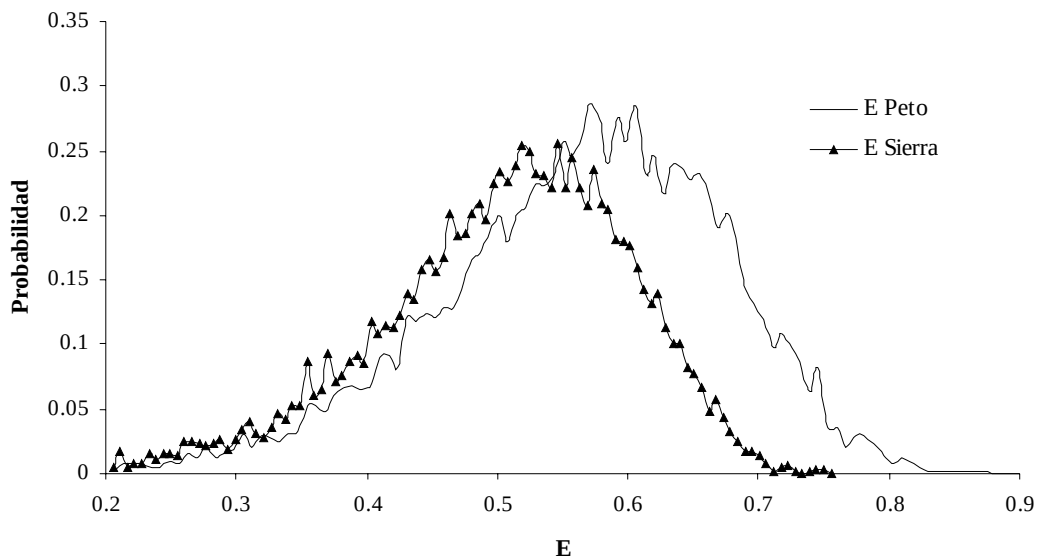
Fig. 6. Distribución de probabilidad aproximada del estimado de E para peto y sierra.
