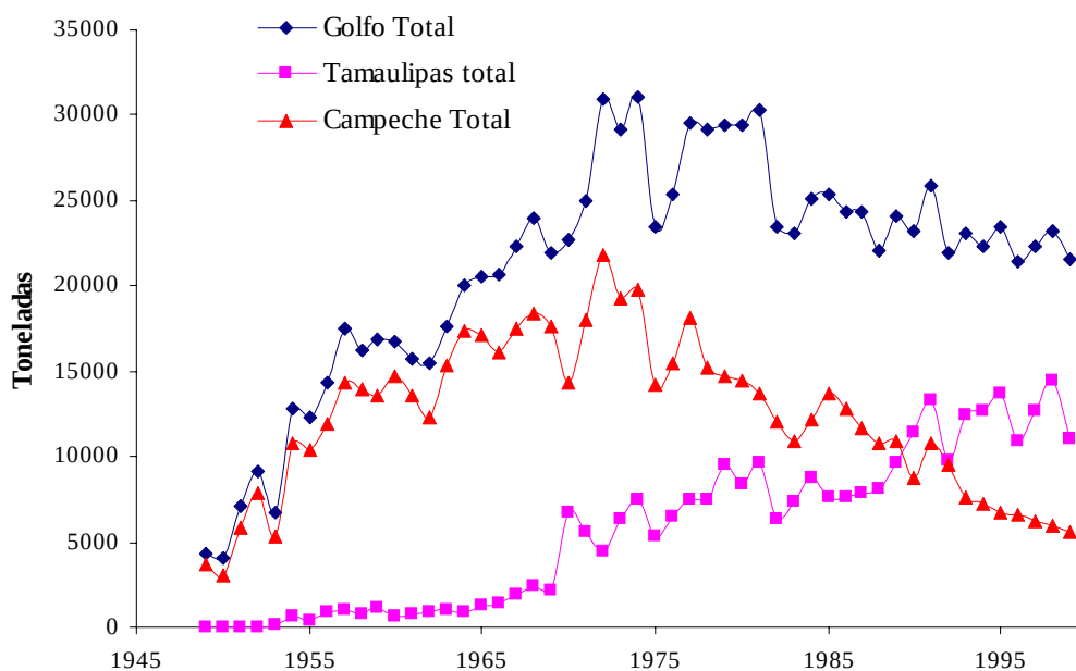
Fig. 4. Evolución de la captura total de camarón en el Golfo de México y en los estados de Tamaulipas y Campeche.
