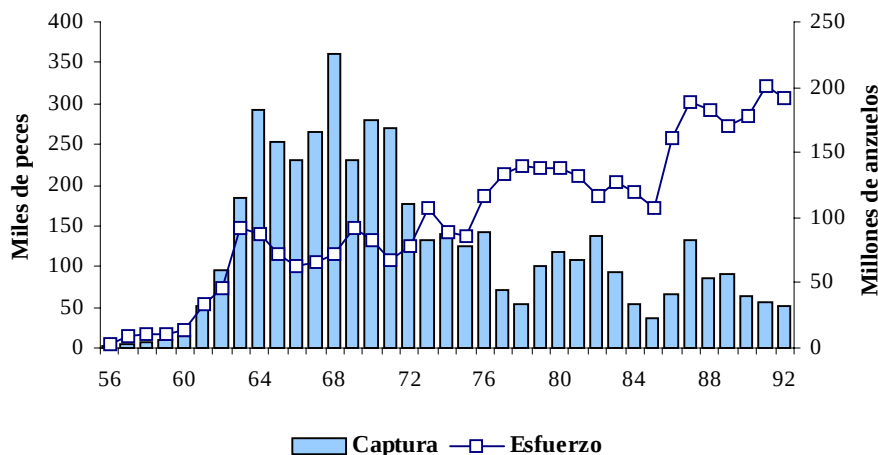
Fig. 5. Captura y esfuerzo de la flota palangrera japonesa en el océano Pacífico oriental, de 1956-92.
