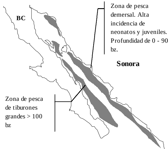
Fig. 6. Principales zonas de captura de tiburón en el Golfo de California.
