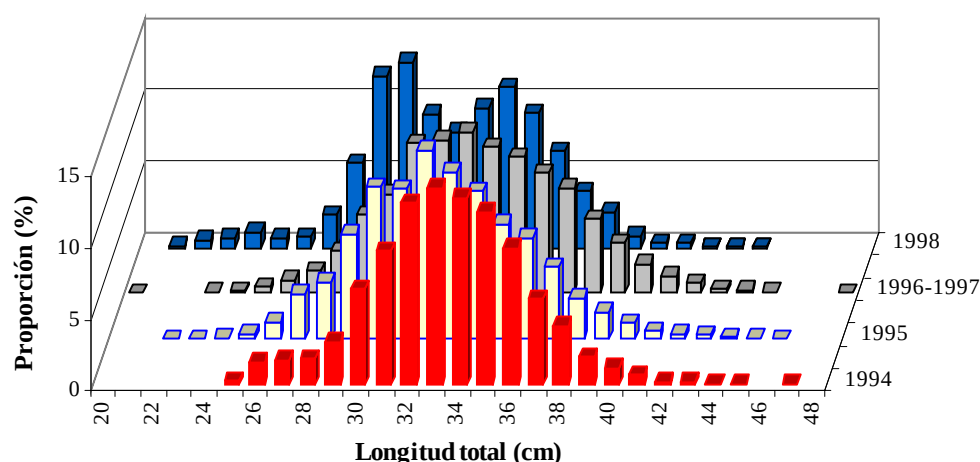
Fig. 8. Distribución de tallas de lisa, Mugil cephalus , en la Laguna Madre, Tamaulipas. 1994-1998.
