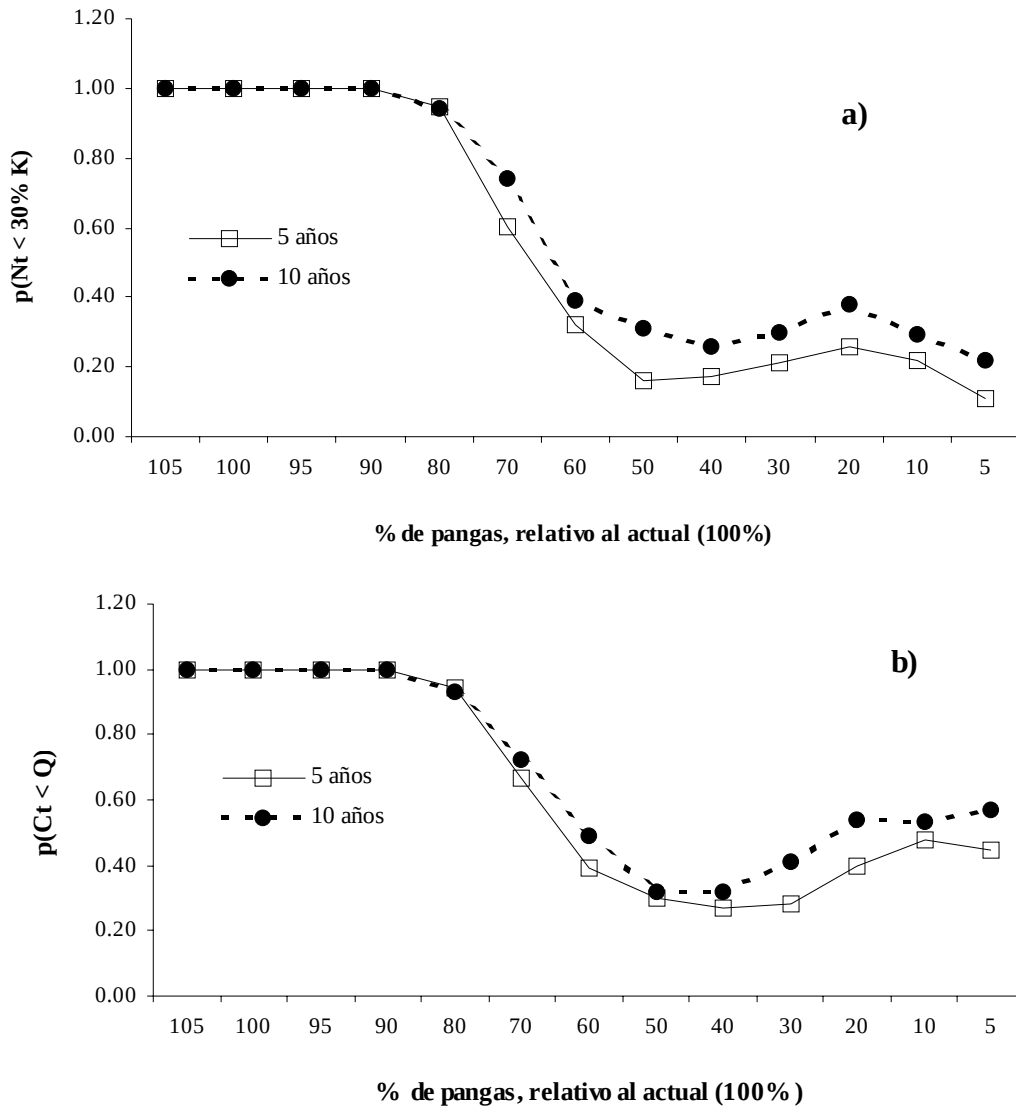
Fig. 6. Probabilidad de que el stock remanente ( N_t ) sea menor a 30% de K (a), y probabilidad de que la captura por temporada ( C_t ) sea menor a la captura óptima ( Q ) correspondiente a un stock de 30% de K (b).
