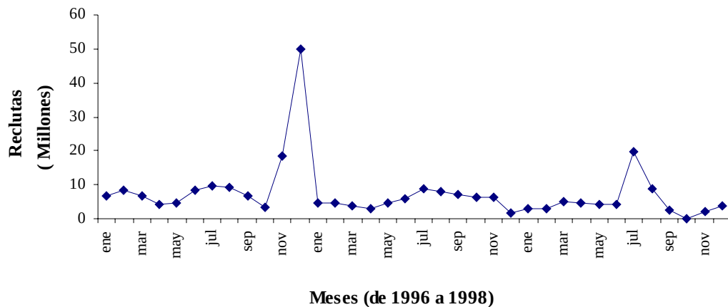
Fig. 23. Número de reclutas estimados por el modelo de enero de 1996 a diciembre de 1998.
