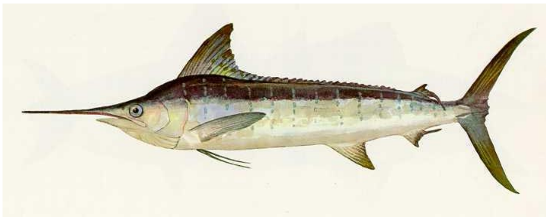
Fig. 1. Marlin Rayado Tetrapturus audax (Philippi, 1887). (Tomado de Joseph, Klawe & Murphy, 1986).
