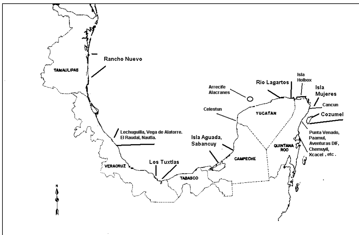
Fig. 2. Principales campamentos de protección de tortuga blanca a lo largo de las costas del Golfo de México.
