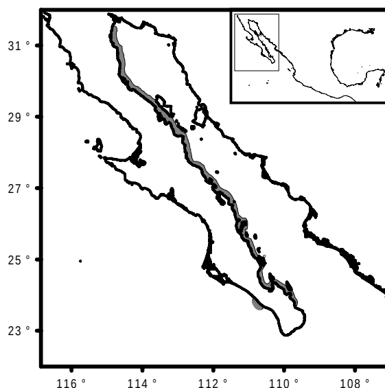
Fig. 1 Distribución de Isostichopus fuscus en la Península de Baja California, México.
