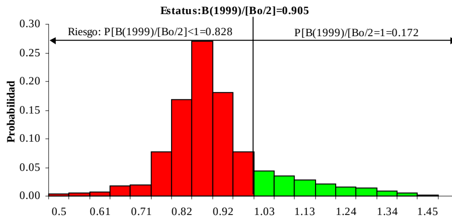
Fig. 15. Estatus del camarón azul, L. stylirostris , en la zona de Mazatlán, Sin. estimada con el modelo dinámico de biomasa de Schaefer.
