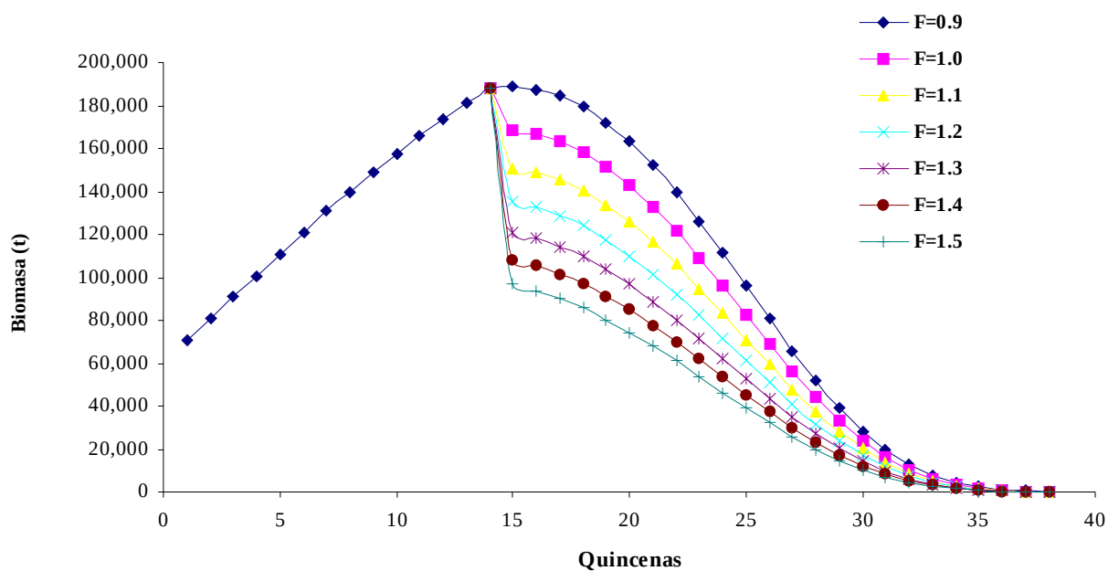
Fig. 7. Diferentes estrategias de explotación de Dosidiscus gigas considerando distintos niveles de mortalidad por pesca.
