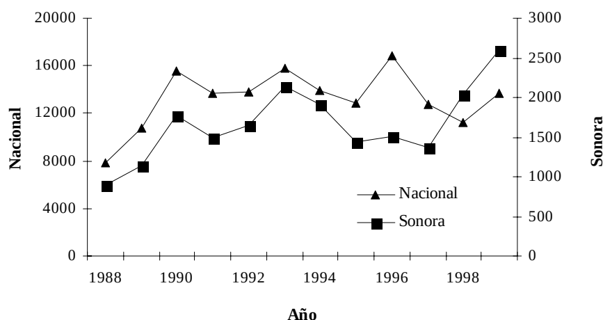
Fig. 4. Captura histórica de sierra (t, peso vivo).
