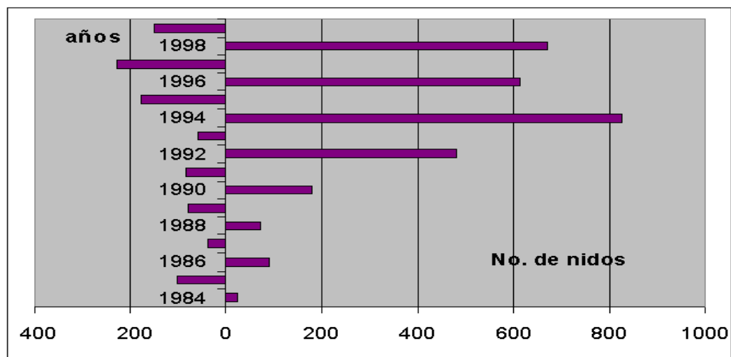
Fig. 5. Comparación de las temporadas de desove de Chelonia mydas en años pares y nones en Campeche, México.
