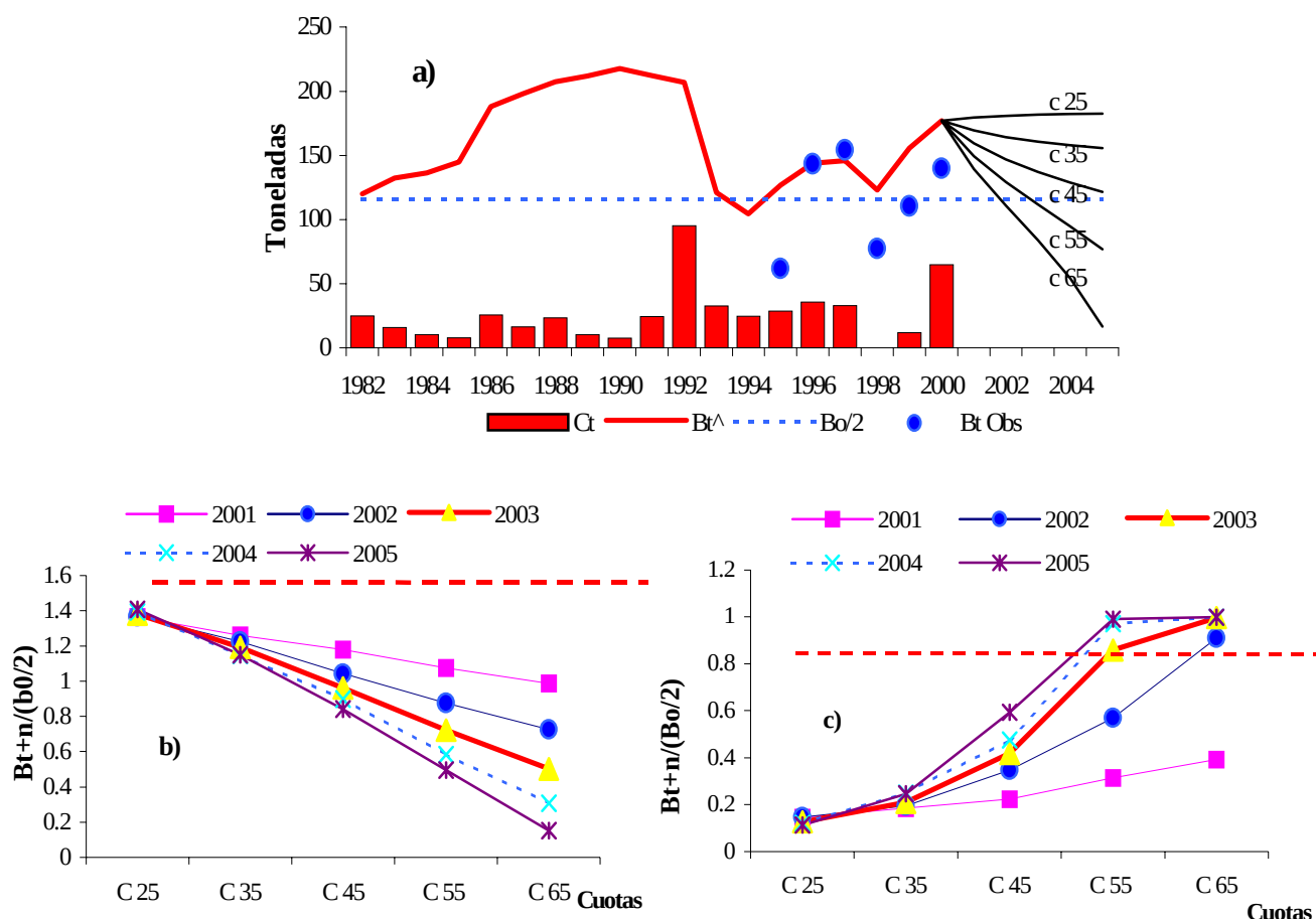
Fig. 11. a) Proyecciones de biomasa, b) Probabilidad del PRO B_{t+n}/(Bo/2) y c) Nivel de riesgo bajo cinco diferentes cuotas de captura para la Zona II.
