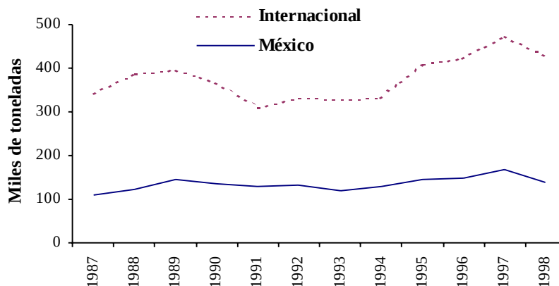
Fig. 3. Tendencia histórica de la captura de atún (varias especies) por la flota atunera internacional y mexicana en el océano Pacífico oriental (SEMARNAP, 1999; CIAT, 1999a).
