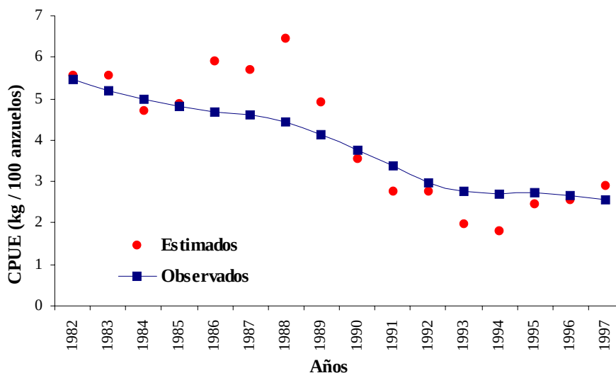
Fig. 10. Ajuste del modelo con la captura por unidad de esfuerzo de la flota cubana (CPUE flota cubana), observada y estimada por el modelo, durante 16 años (1982 – 1997).
