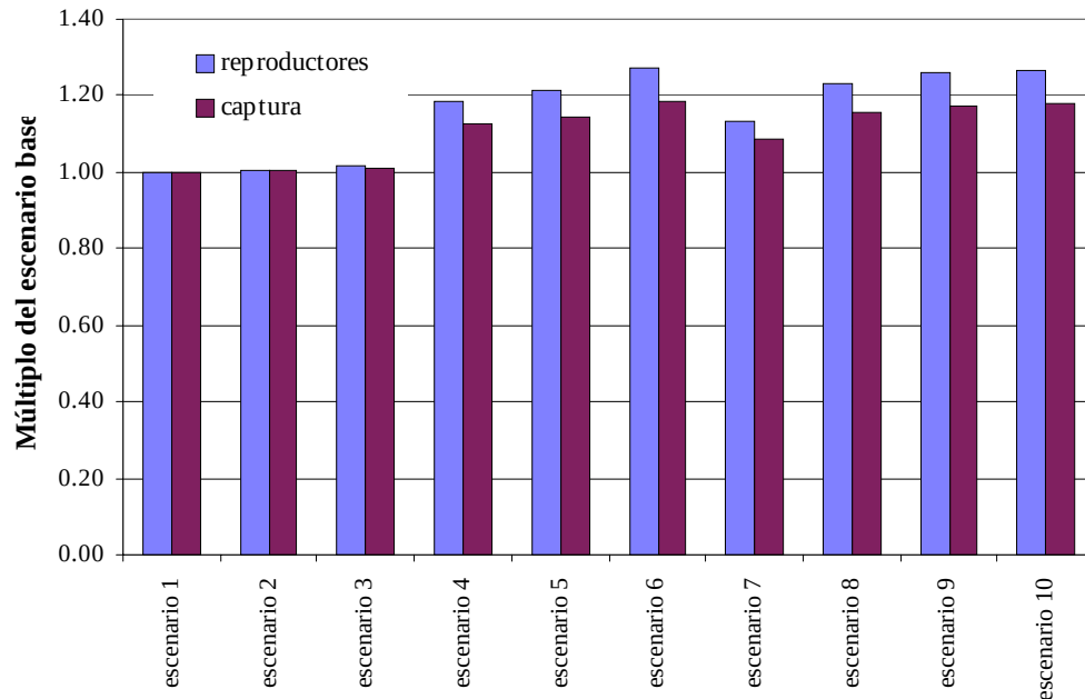
Fig. 25. Captura y abundancia relativas con diferentes alternativas de veda
