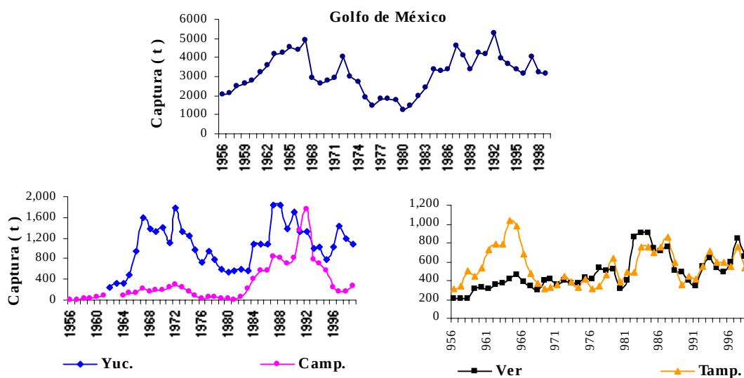
Fig. 3. Comportamiento histórico de las capturas de huachinango obtenidas en el Golfo de México de 1956 a 1999 (SEMARNAP Delegaciones Federales en el Golfo de México).
