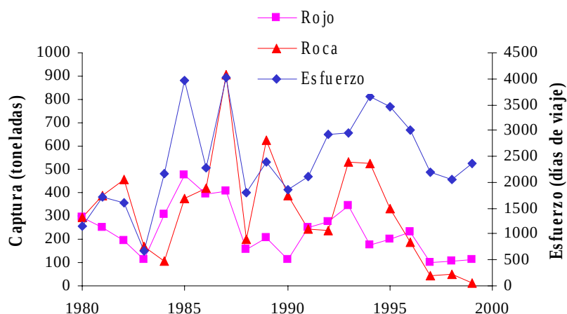
Fig. 14. Tendencia histórica de las capturas de camarón y esfuerzo en Contoy.
