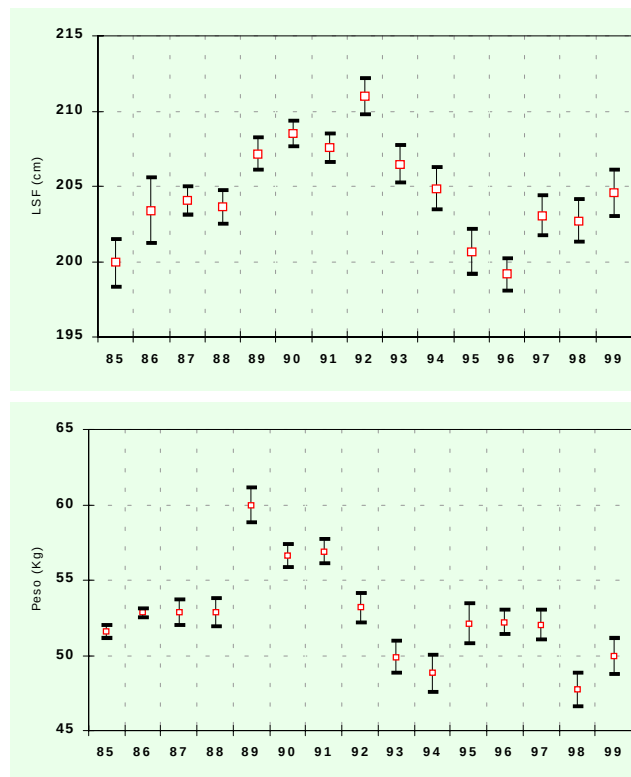
Fig. 4. Variación anual de tallas (a) y pesos (b) medios de marlin rayado, e intervalos de confianza respectivos, durante los años de 1985 a 1999.
