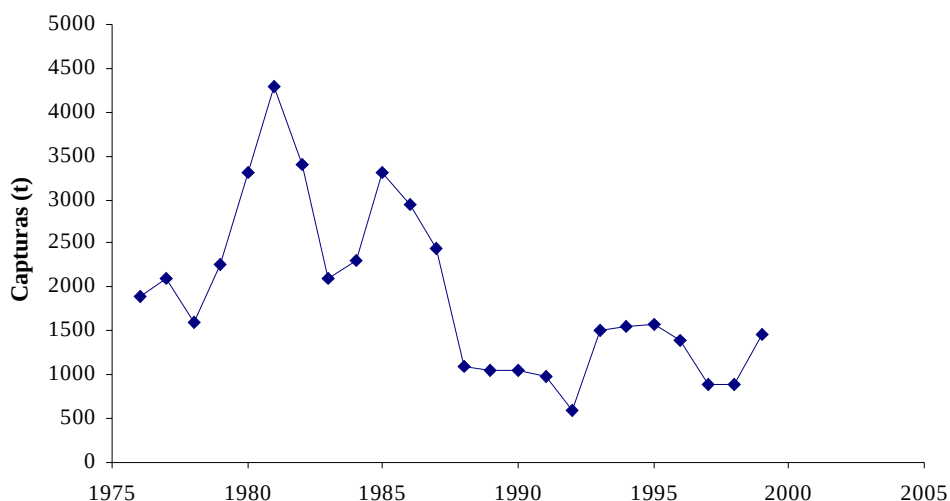
Fig. 2. Captura de lisa en Sinaloa, 1976-1999. Fuente: Delegación Federal de Sinaloa.
