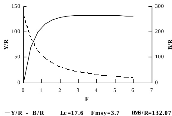
Fig. 3. Rendimiento y biomasa por recluta de Oreochromis aureus en función de la tasa de mortalidad por pesca.
