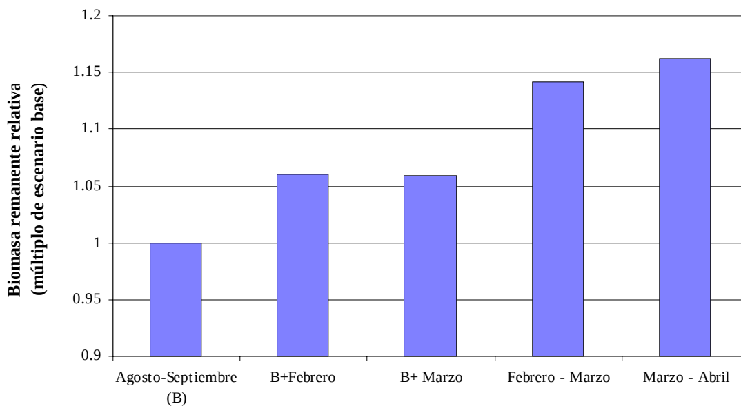
Fig. 29 . Biomasa Remanente relativa obtenida bajo los diferentes escenarios de veda.
