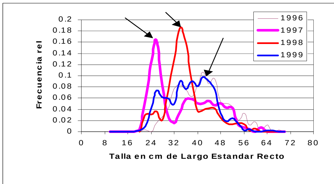
Fig. 3. Distribución de frecuencias registradas frente a la Reserva de Río Lagartos. Las flechas marcan la progresión anual de una cohorte que se reclutó a la vida demersal en 1997.
