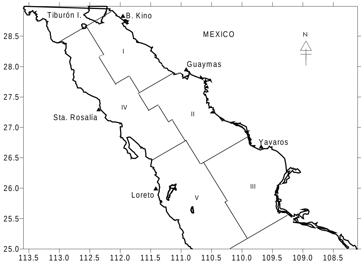
Fig. 3. Distribución de los cinco estratos seleccionados en el Golfo de California.
